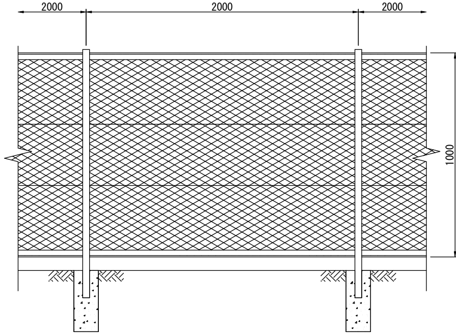
正面図 S=1:20
