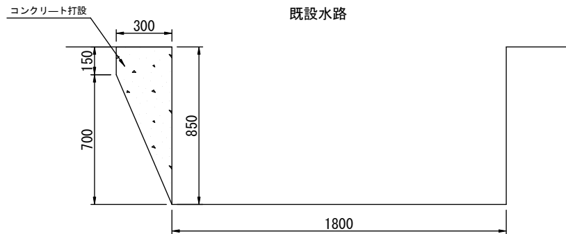
断面補修 標準断面図 S=1:20
