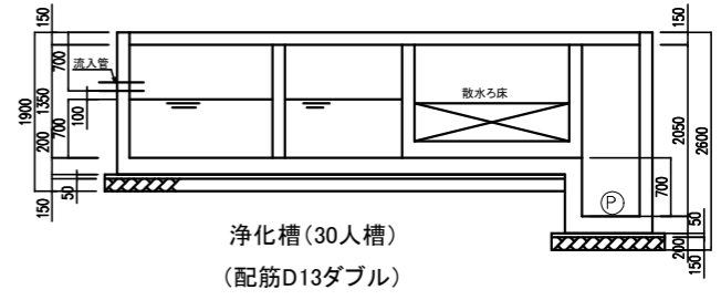
断面図 S=1:50
