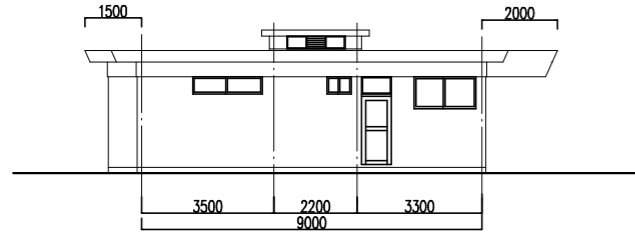
西立面図 S=1:100
