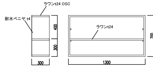
台所棚詳細 S=1:20
