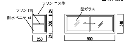
事務室 ベット上部棚詳細 S=1:20
