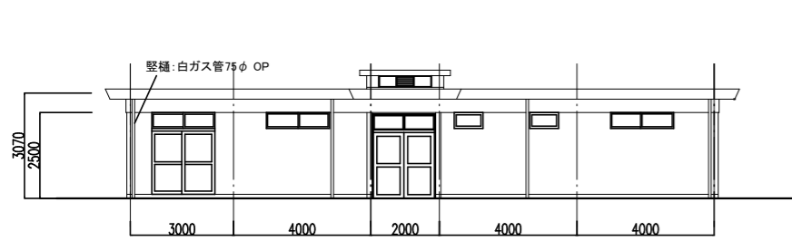
北立面図 S=1:100
