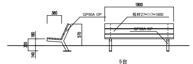
ベンチ詳細図 S=1:30
