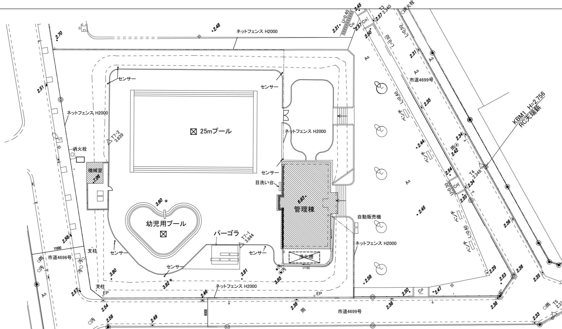
配置図 S=1:200
