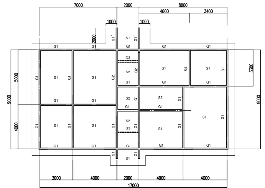
梁伏図 S=1:100
