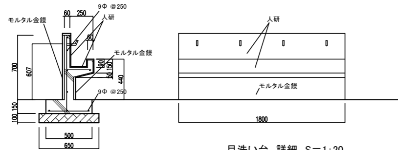
目洗い台 詳細 S=1:20
