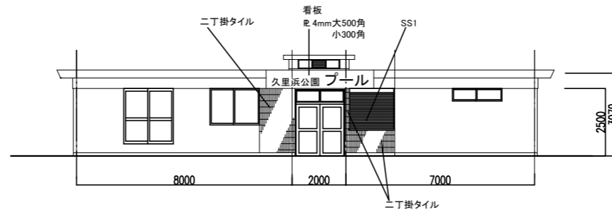
南立面図 S=1:100
