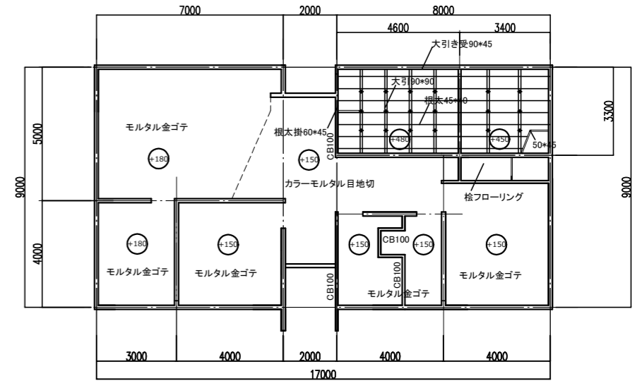
床伏図 S=1:100
