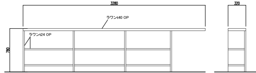
コート預り所カウンター詳細 S=1:20
