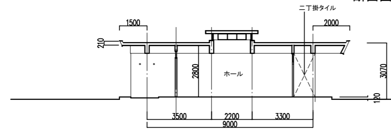
B-B 断面図 S=1:100
