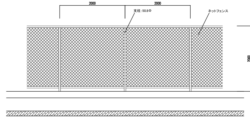
外柵 ネットフェンス 詳細図 S=1:30
