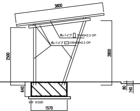
パーゴラ詳細図 S=1:50
