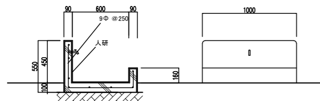
足洗い場 詳細 S=1:20
