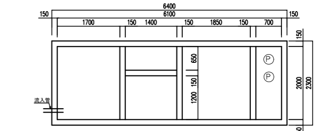
平面図 S=1:50
