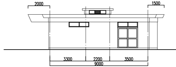
東立面図 S=1:100
