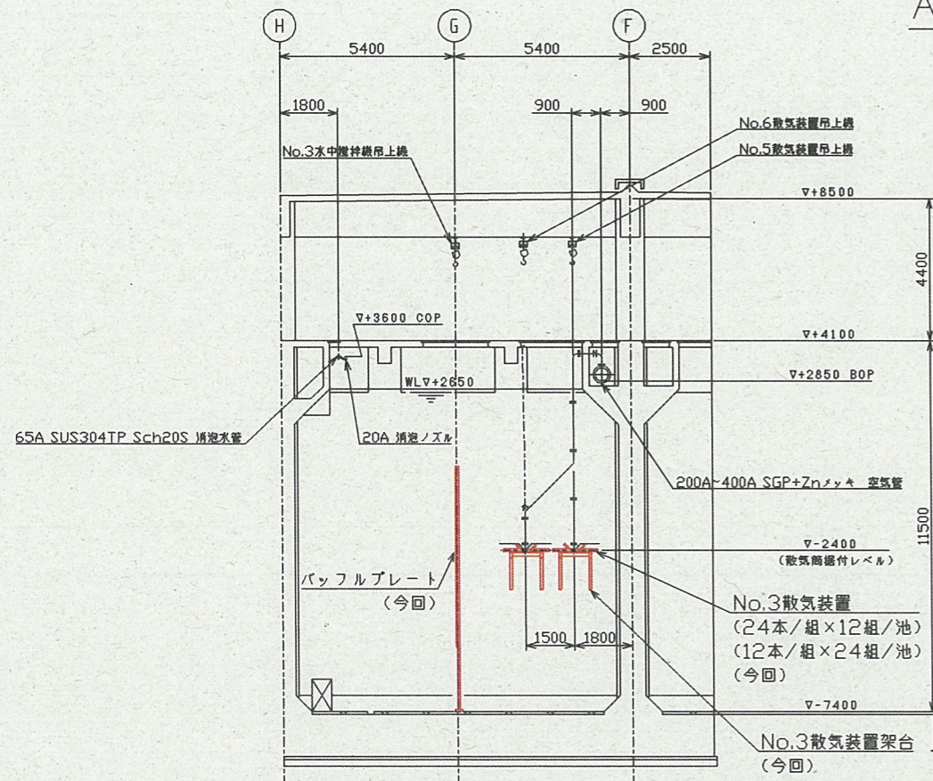
B-B断面図 (S = 1 / 100)
