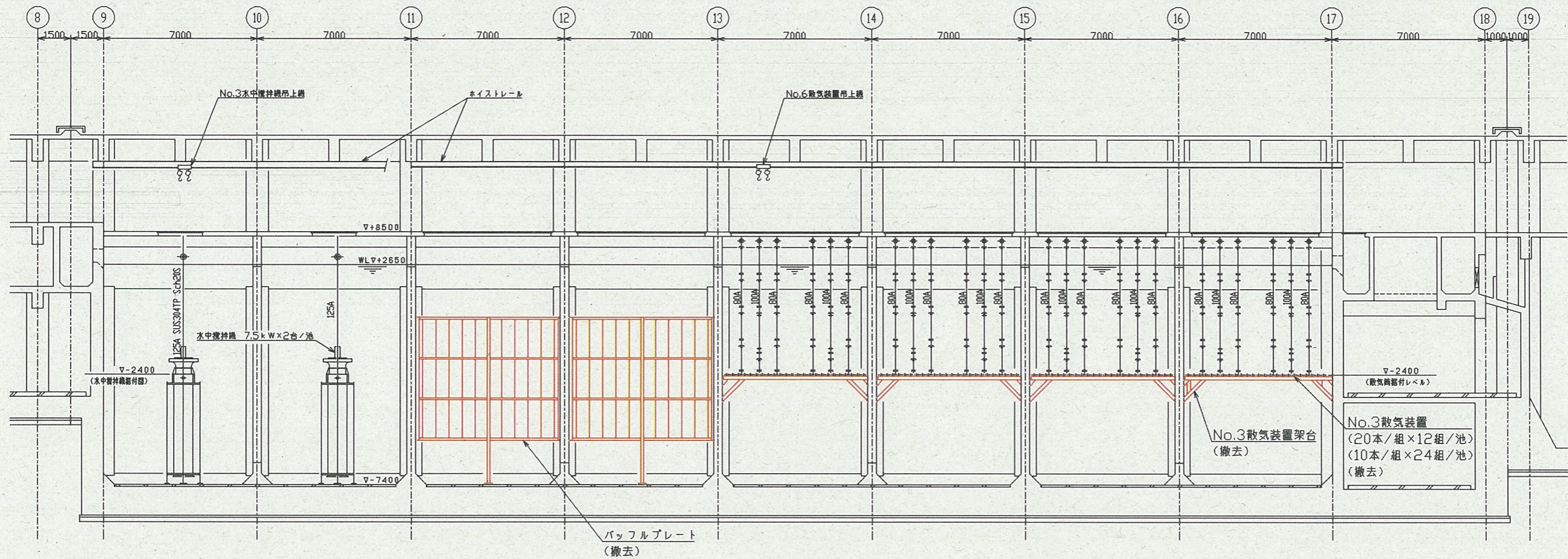
A - A 撤去断面図 (S = 1 / 100)
