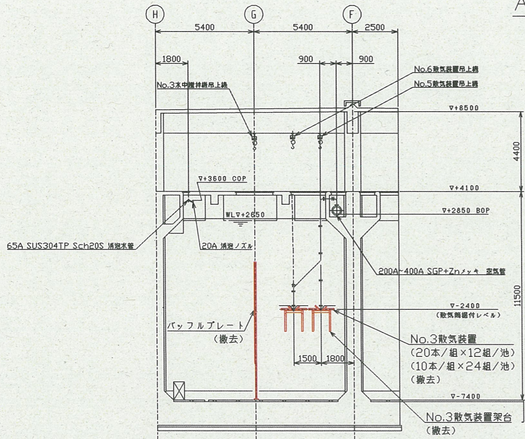
B - B 撤去断面図 (S = 1 / 100)
