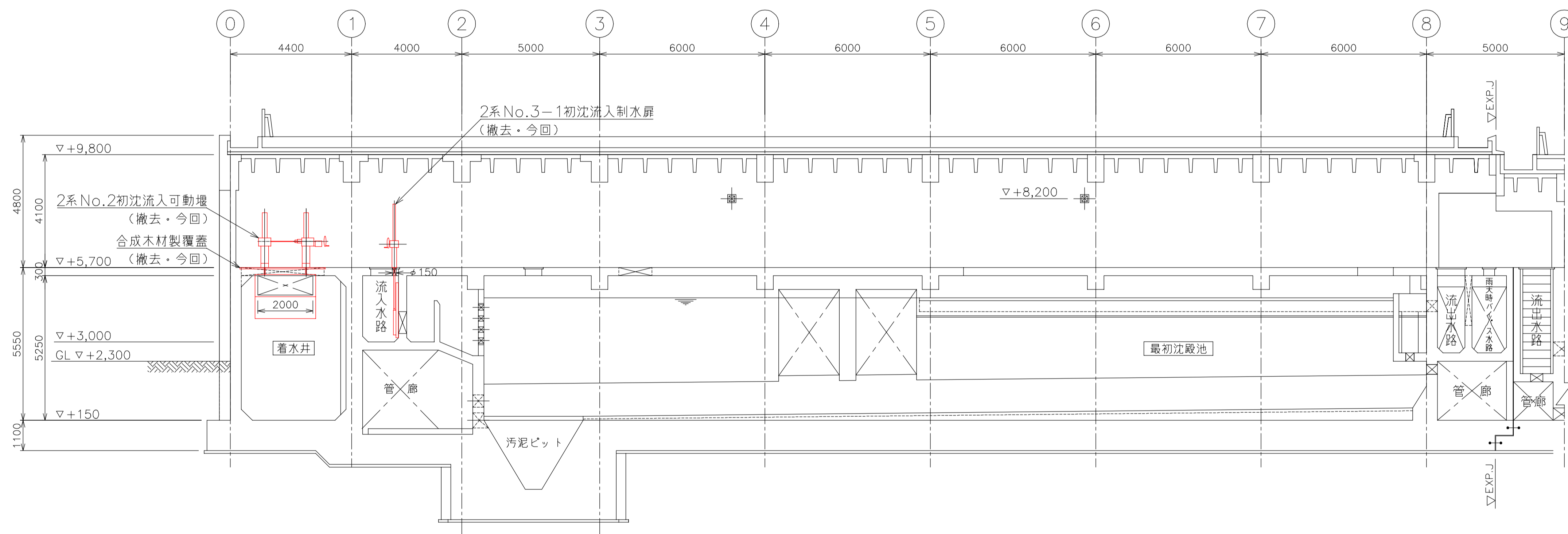
A-A 断面図 S=1/100
