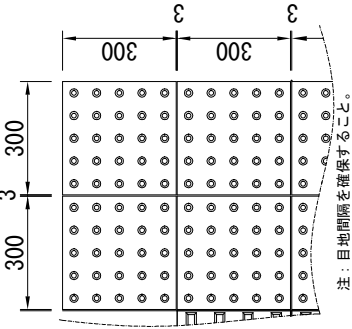
貼付式点字 割付平面図
