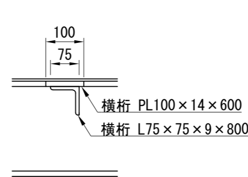
1-1断面 1:10
