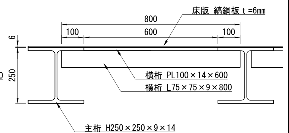
2-2断面 1:10
