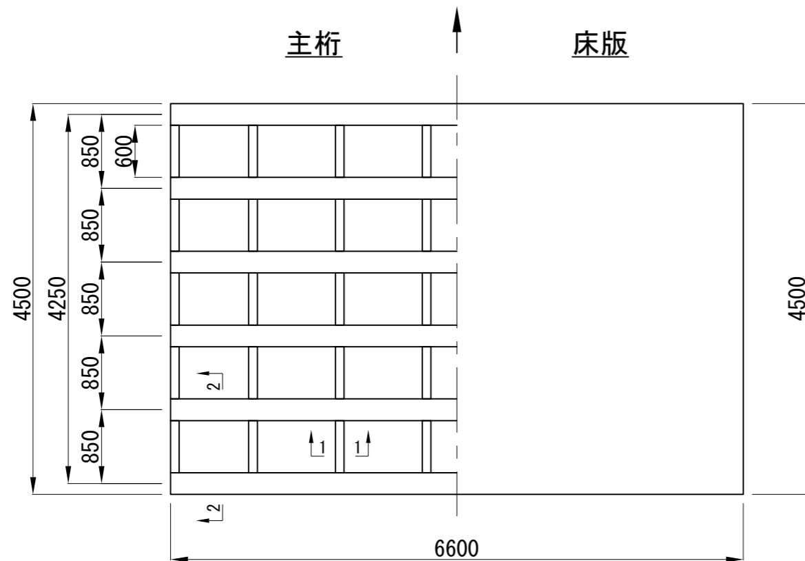
平面図 1:60
