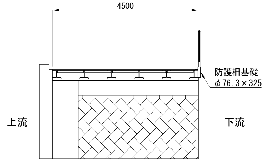
上部工断面図 1:60
