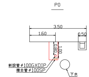
断面図 S=1/50
