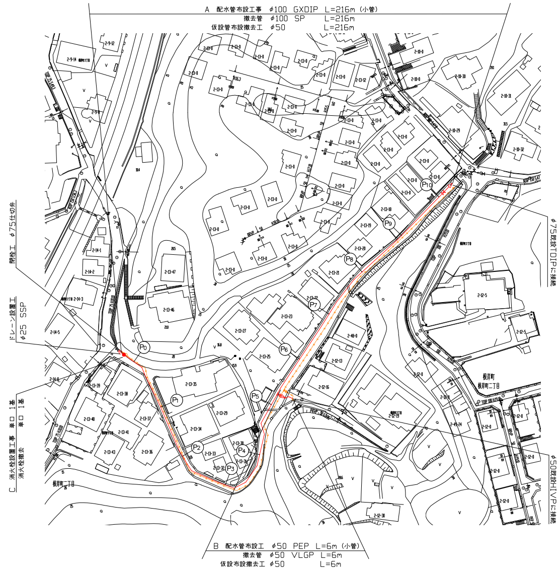
平面図 S=1/500
