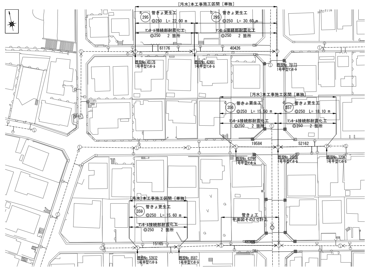
平面図 1-2 S=1:300
