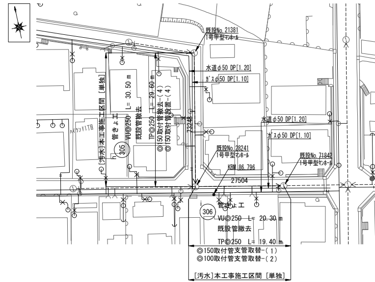
平面図 2-1 S=1:300
