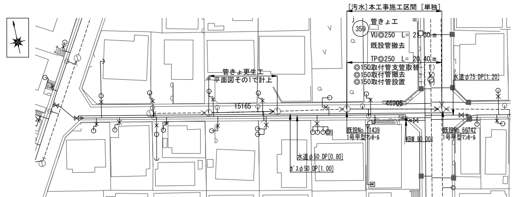
平面図 2-2 S=1:300
