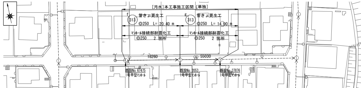
平面図 1-2 S=1:300
