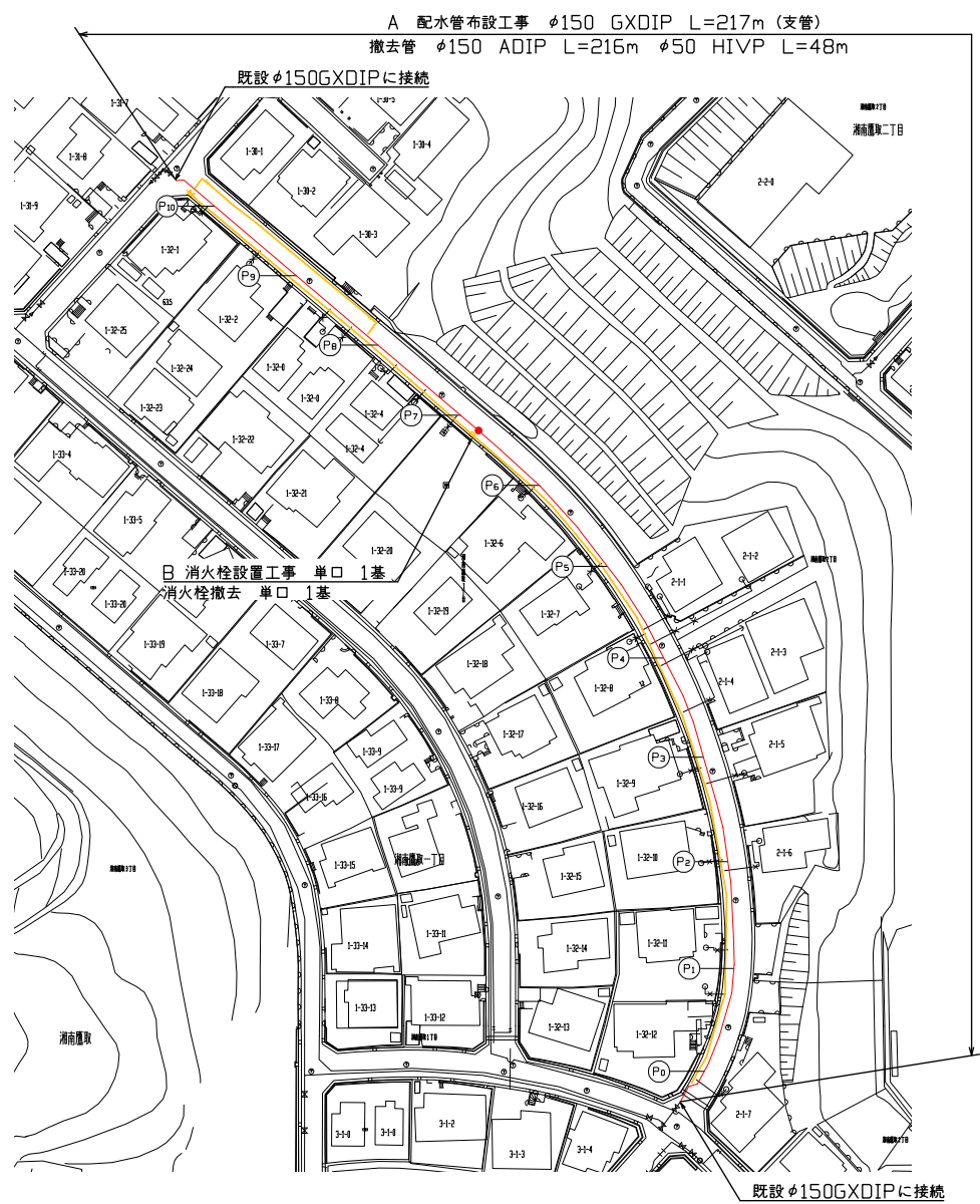
平面図 S=1:500
