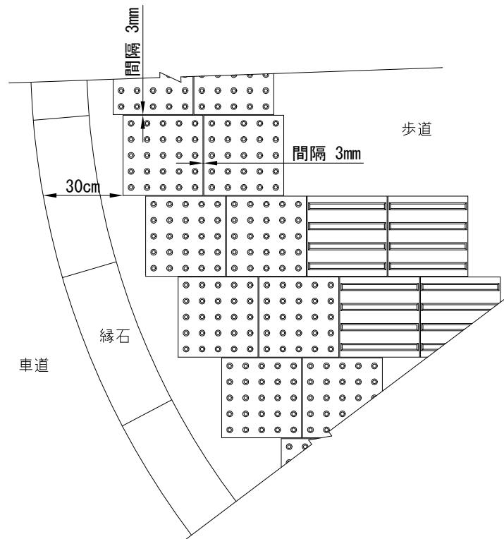
貼付平面図 1:20
