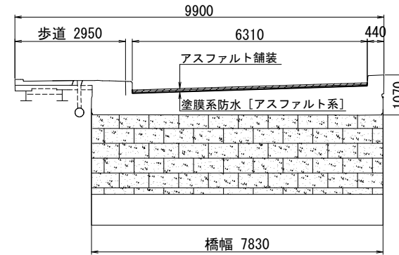
横断面図
