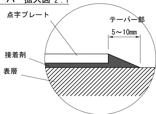
テーパー拡大図 2:1
