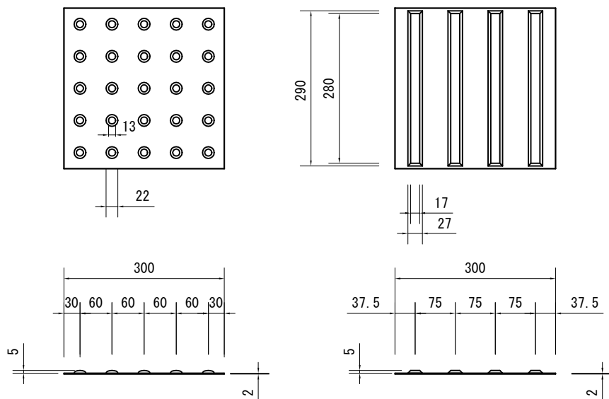
断面詳細図 1:1
