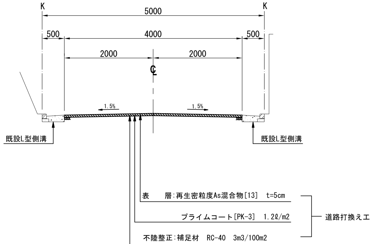
No.10付近 B-B断面
