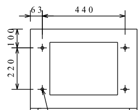
(前面) アンカーボルト取付用穴
