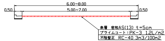
標準横断面図
