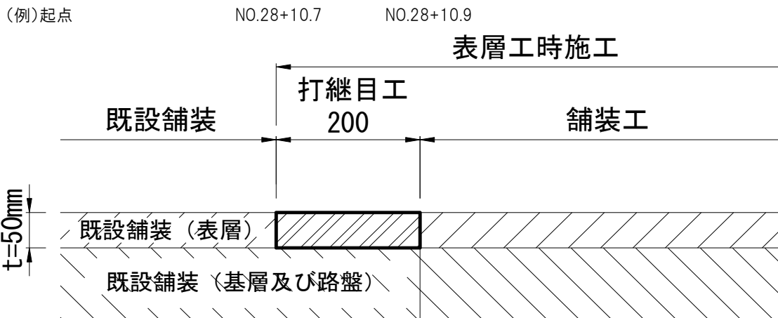
打継目工概略図
