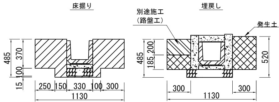
U型側溝 (U240)
