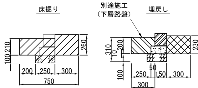
地先境界ブロック
