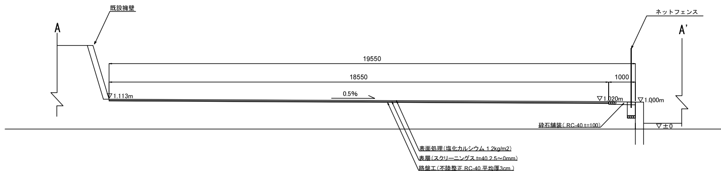
A-A' 断面図 1/100
