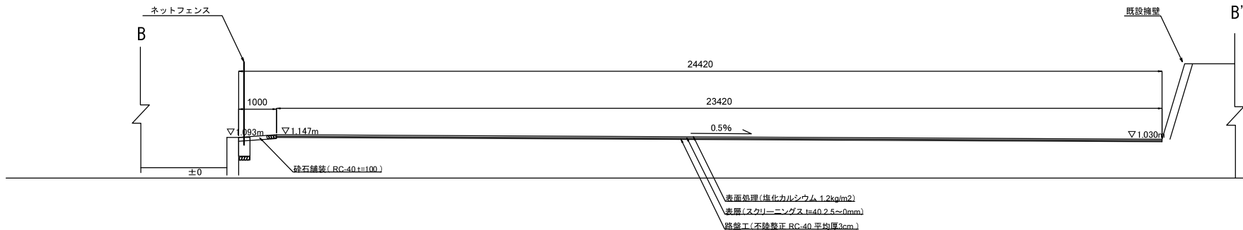
B-B' 断面図 1/100
