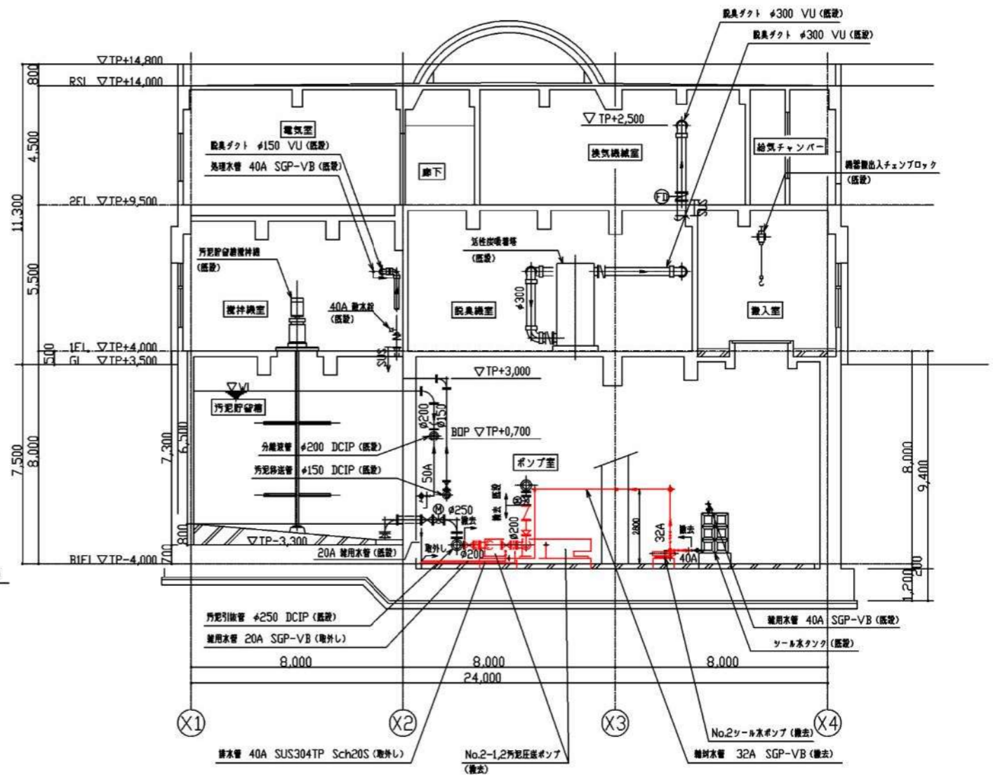
A-A断面図 (S=1/100)
