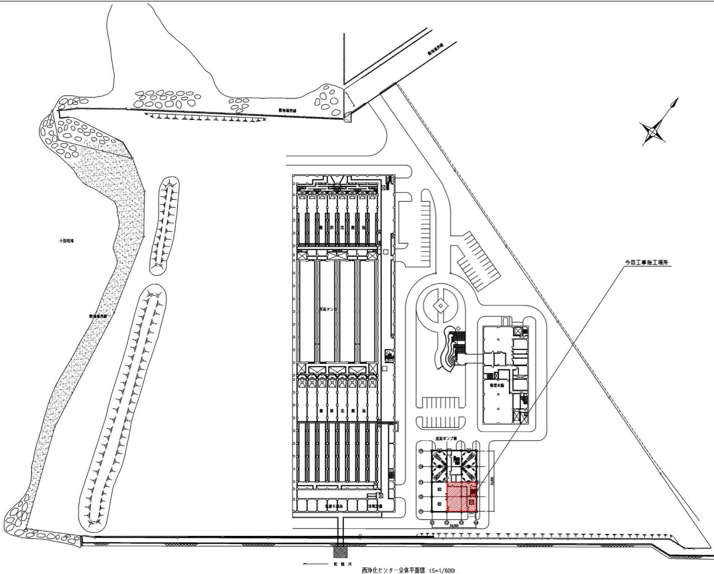
西浄化センター全体平面図 (S=1/600)
