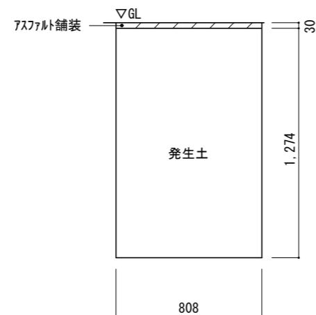
撤去後 東電引込側 高压配管路掘削断面図 1:30
