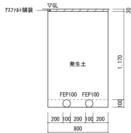
施工後 UGS 2次側 高圧配管路掘削断面図 1:30
