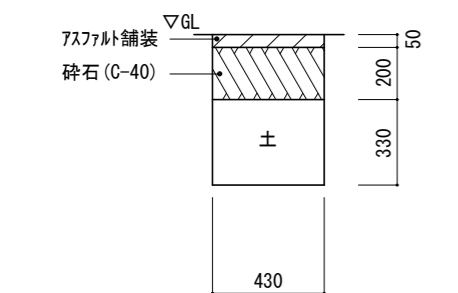
施工前 別途監視カメラ・スピーカー用 配管路掘削断面図 1:30
