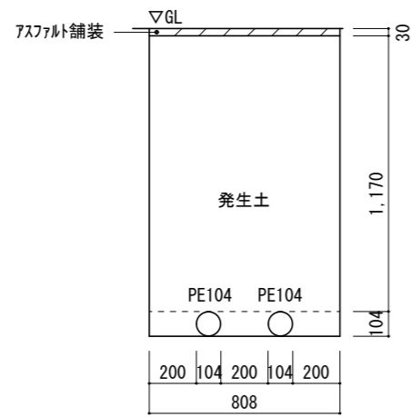
施工後 東電引込側 高圧配管路掘削断面図 1:30
