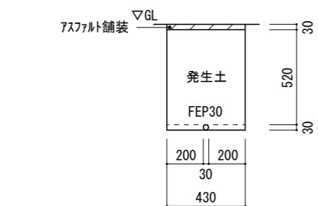
施工後 別途監視カメラ・スピーカー用 配管路掘削断面図 1:30
