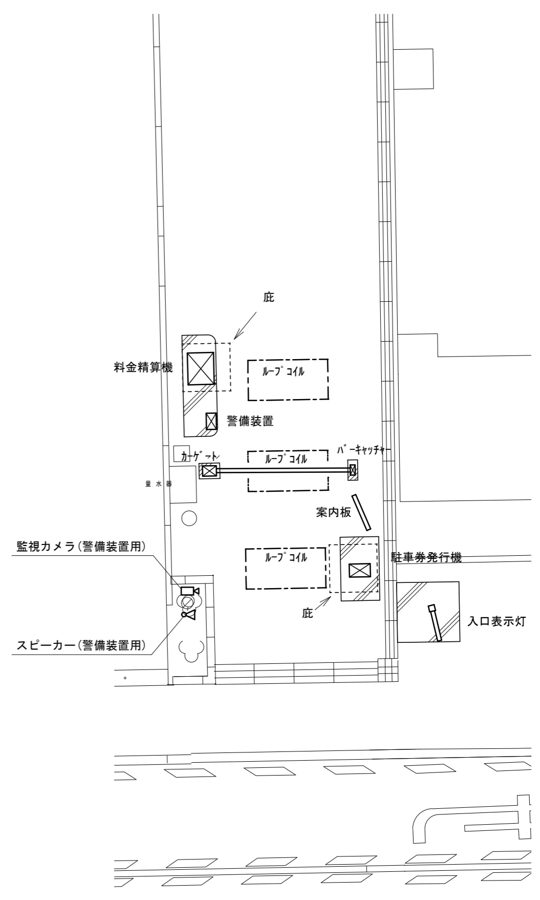
1階 移設・撤去図 1:100
