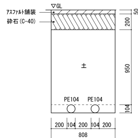
撤去前 東電引込側 高压配管路掘削断面図 1:30
