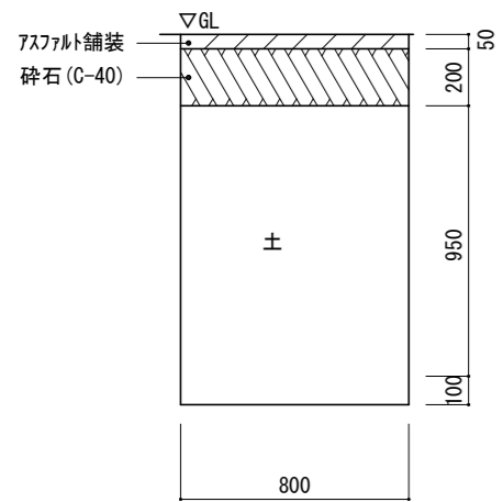
施工前 UGS 2次側 高圧配管路掘削断面図 1:30
