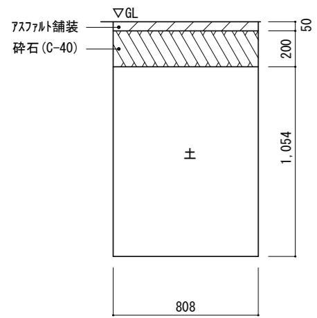
施工前 東電引込側 高圧配管路掘削断面図 1:30
