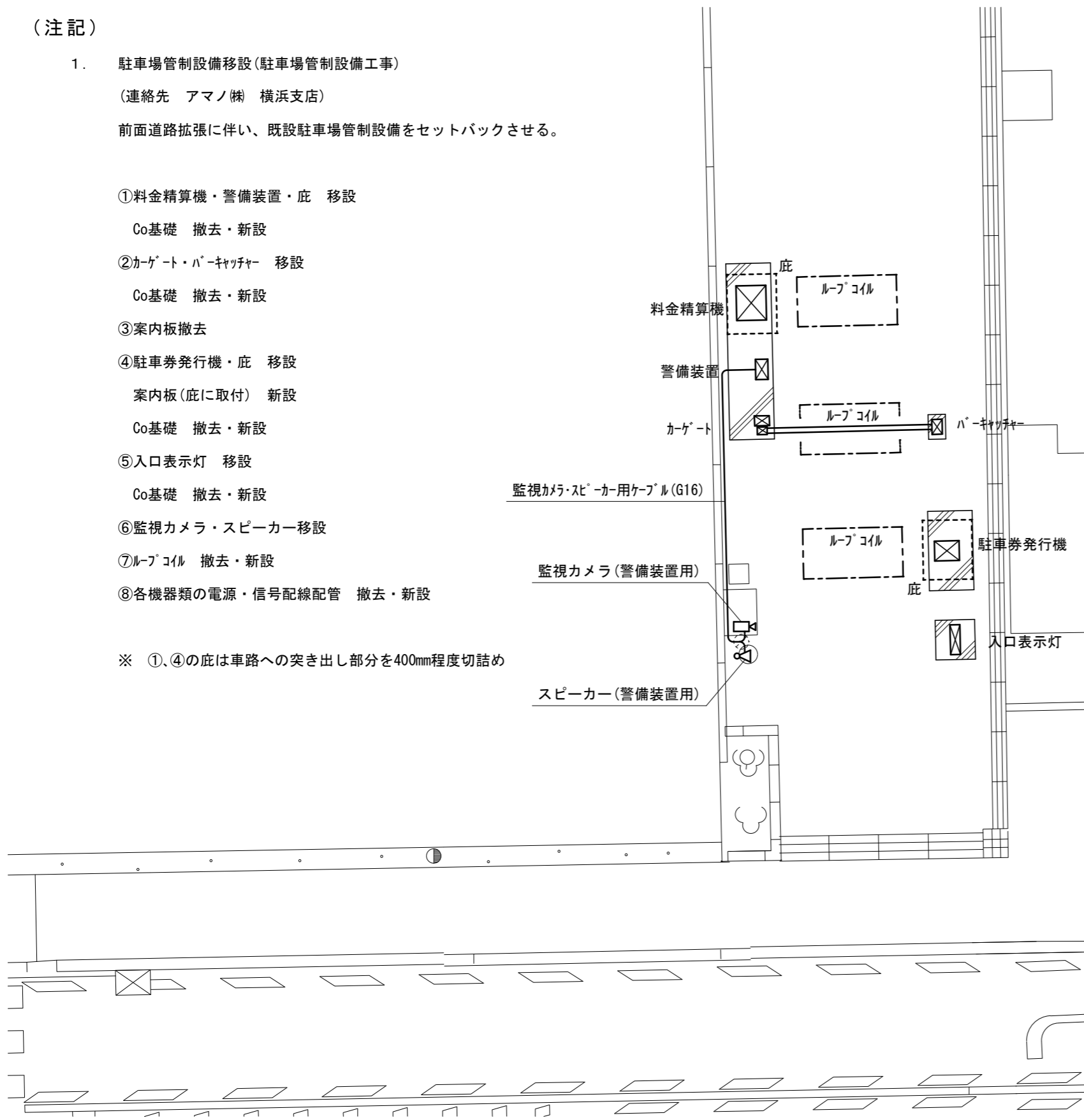
1階 移設・新設図 1:100
