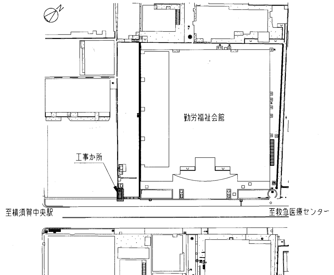
配置図 1: 600
