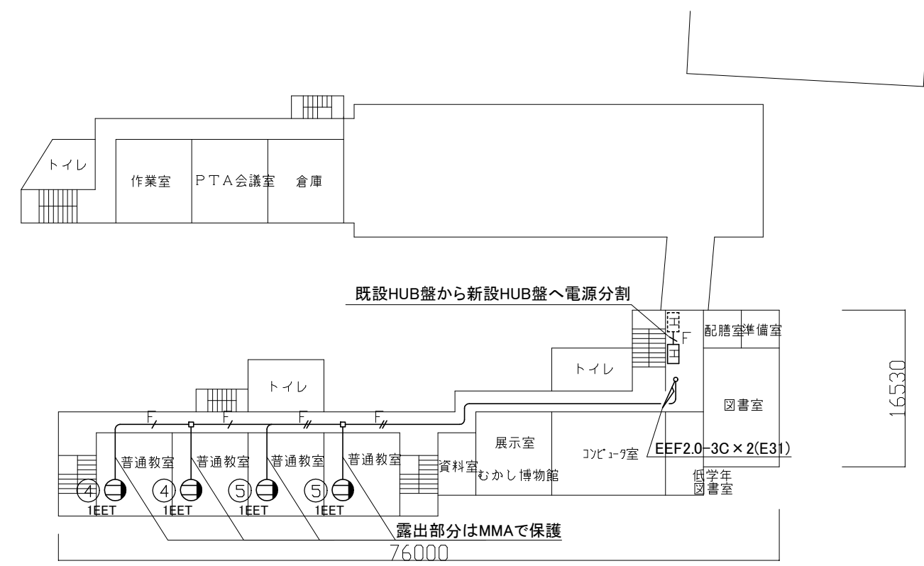
3階配線図 1/400
