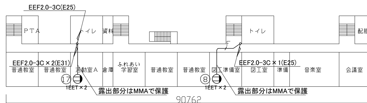
3階配線図 1/400
