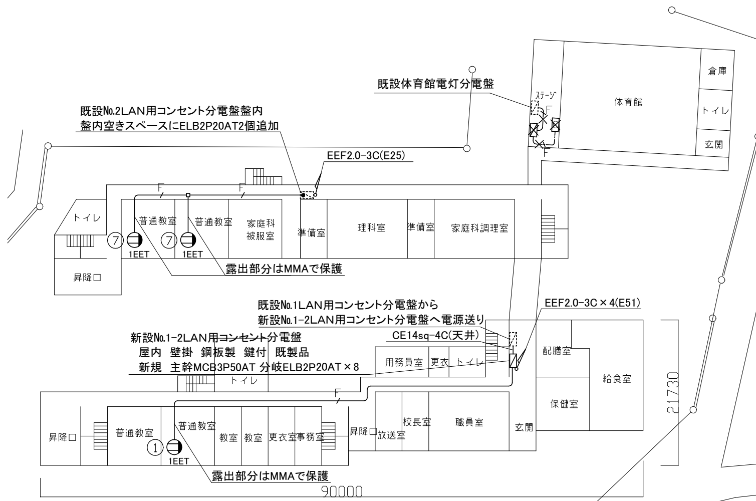
配置図・1階配線図 1/400
