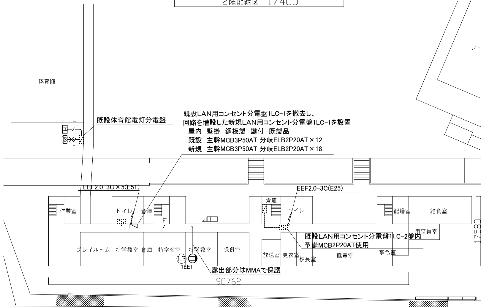
配置図・1階配線図 1/400
