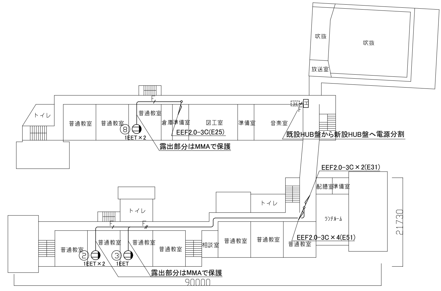
2階配線図 1/400
