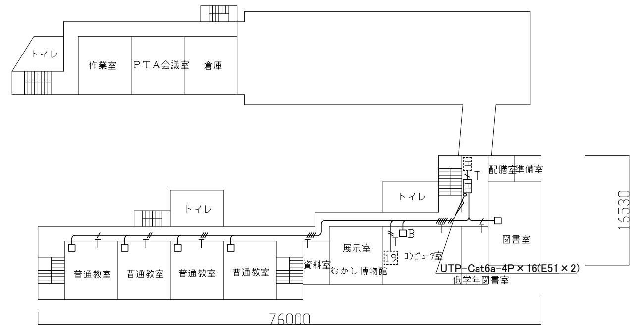
3階配線図 1/400
