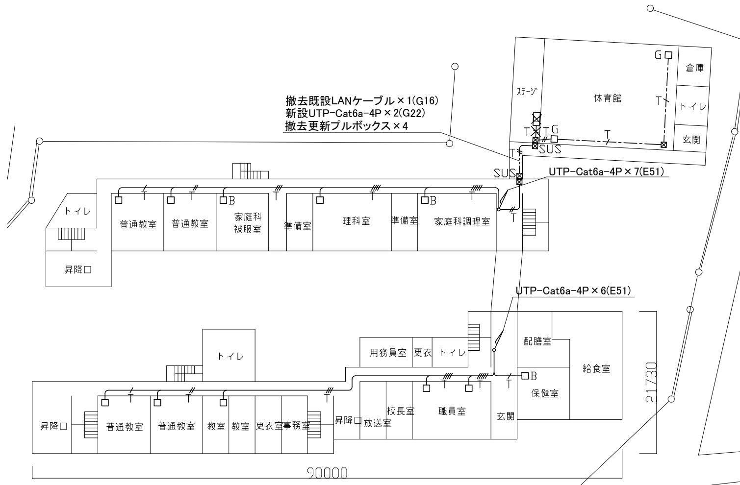
配置図・1階配線図 1/400
