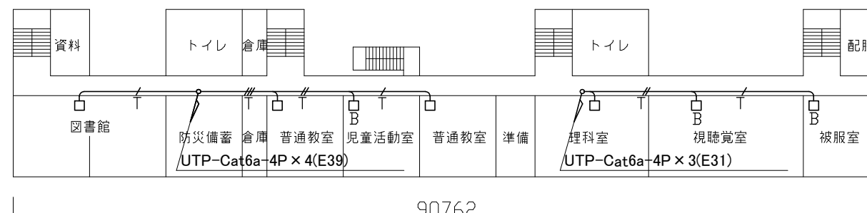
4階配線図 1/400
