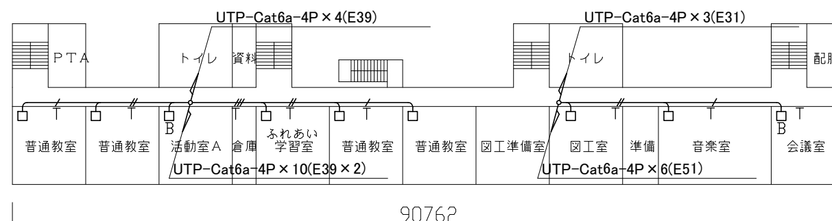
3階配線図 1/400
