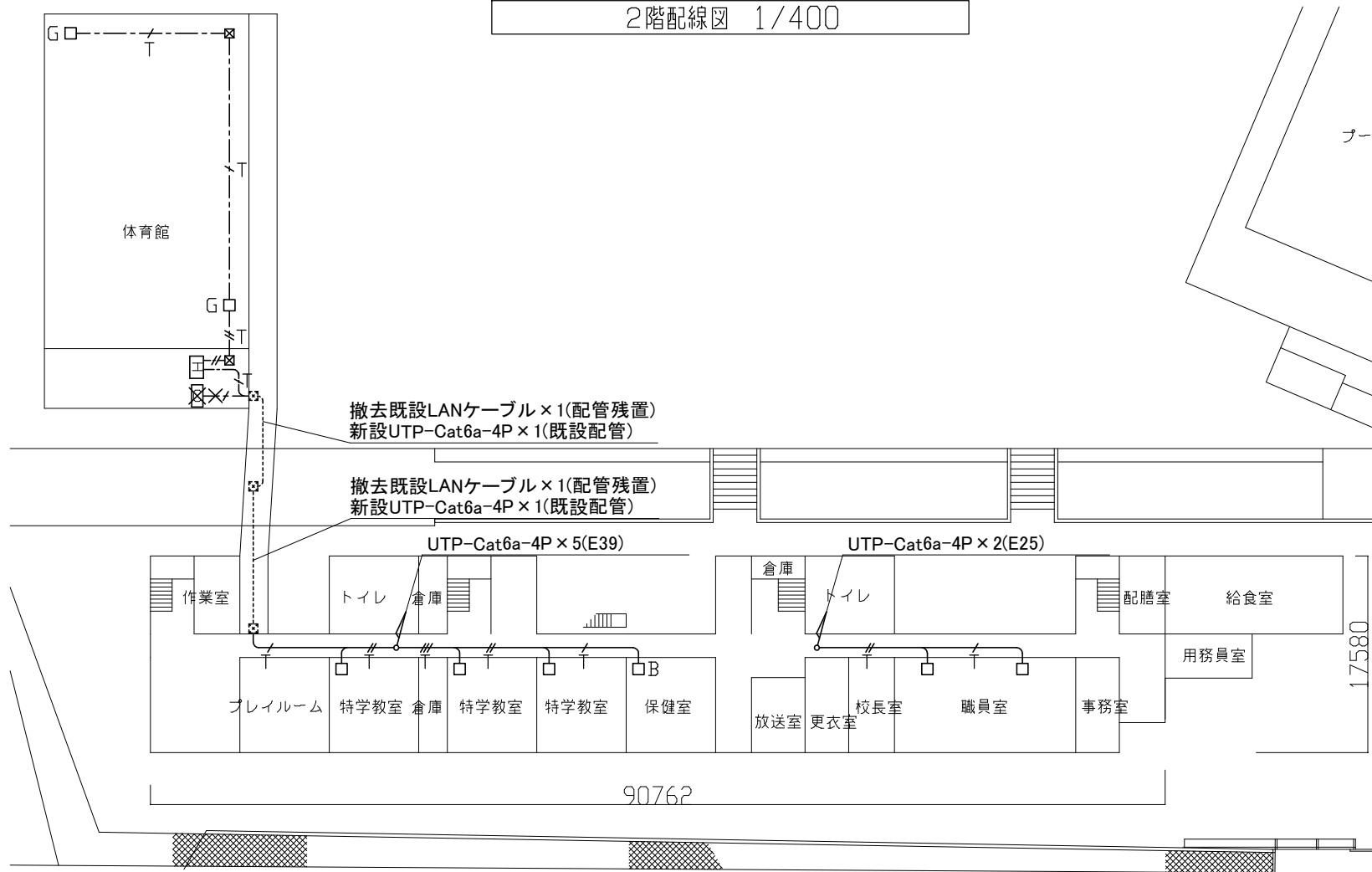
配置図・1階配線図 1/400
