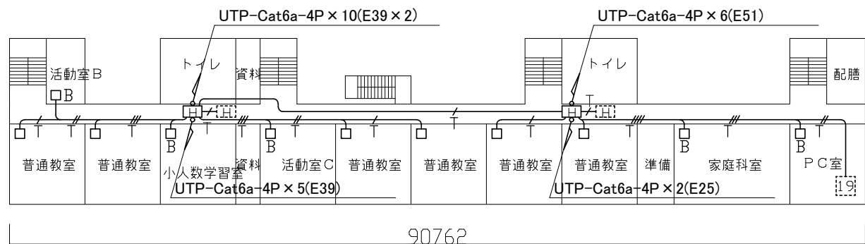
2階配線図 1/400
