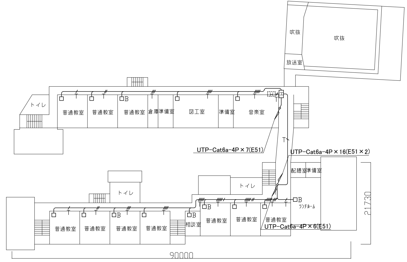
2階配線図 1/400
