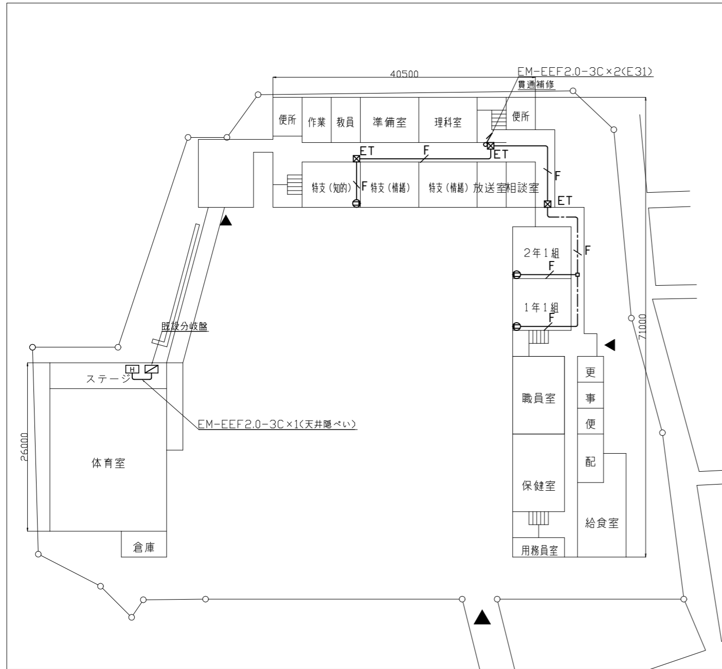
1階電源配線図 1:600
