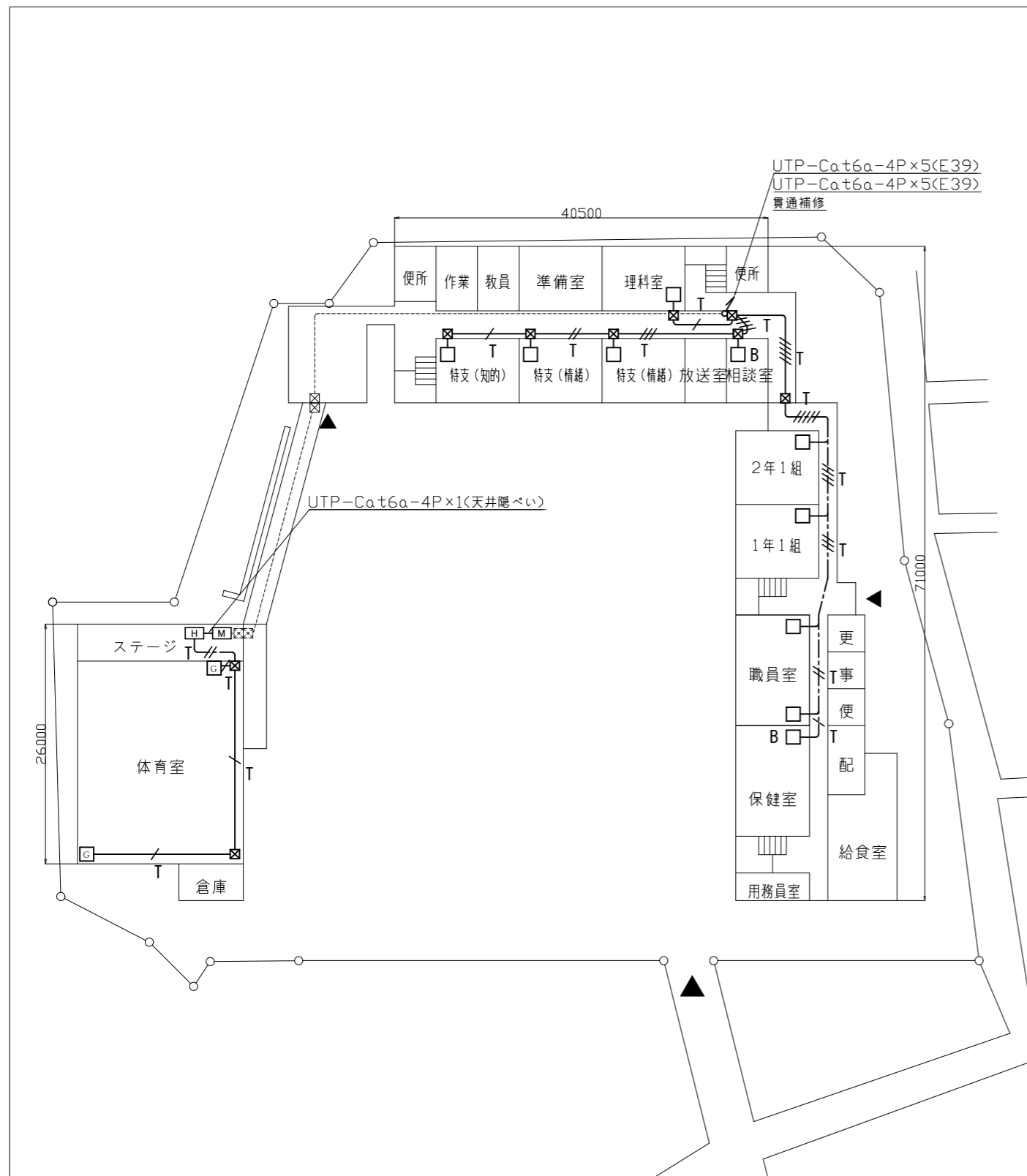
1階LAN配線図 1:600
