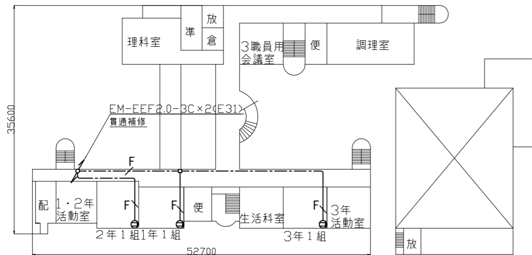
2階電源配線図 1:600
