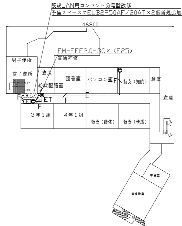
2階電源配線図 1:600
