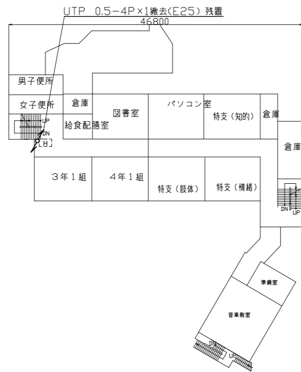
2階LAN配線撤去図 1:600
