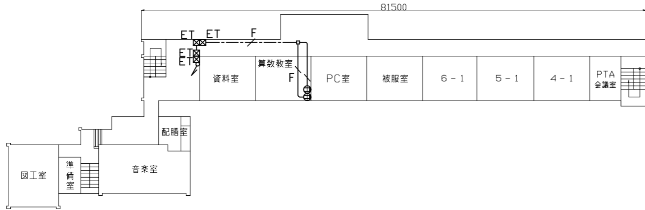
3階電源配線図 1:600
