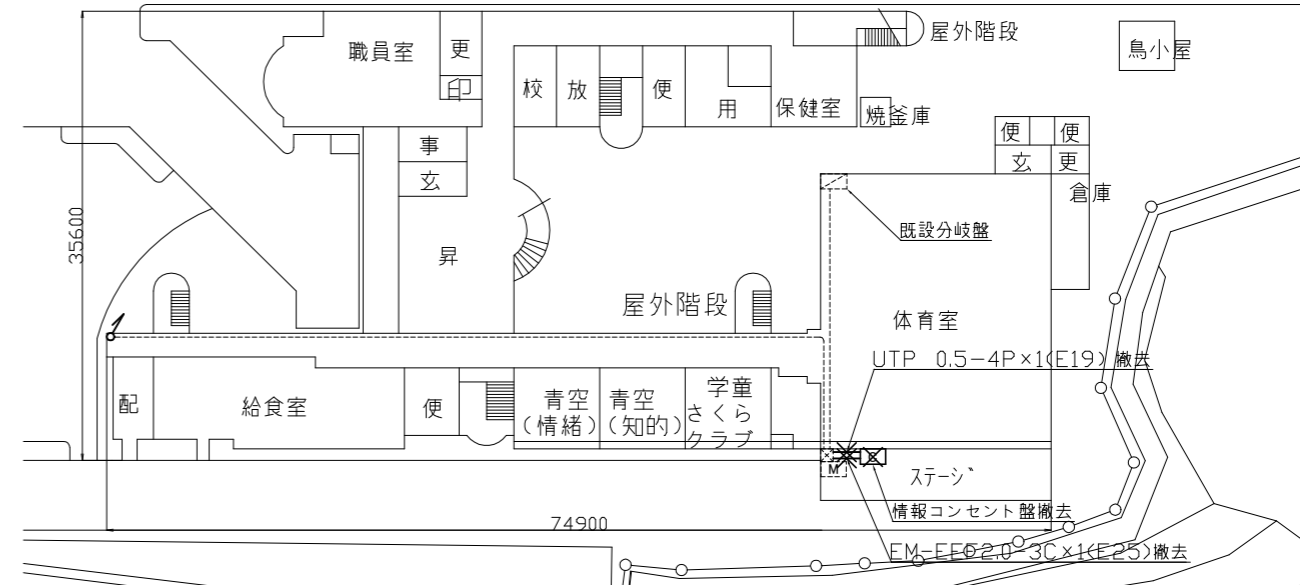
1階LAN・電源配線撤去図 1:600
