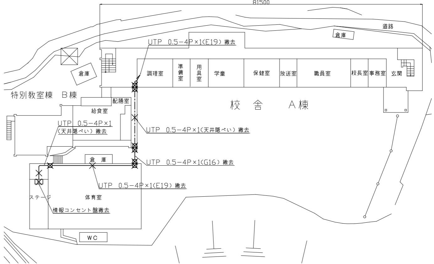
1階LAN配線撤去図 1:600
