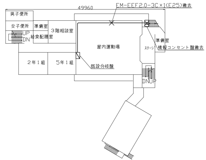
3階電源配線撤去図 1:600
