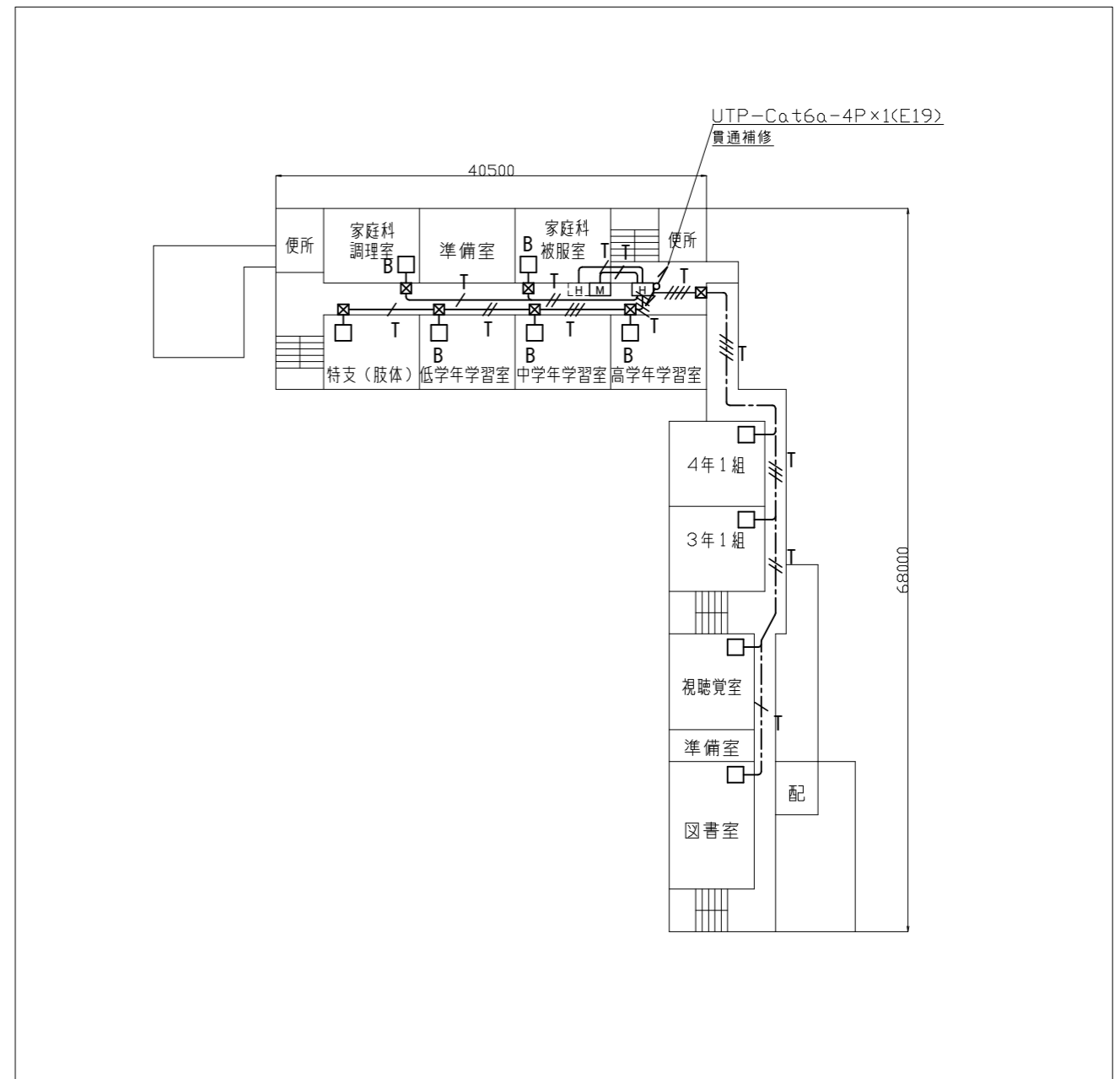
2階LAN配線図 1:600
