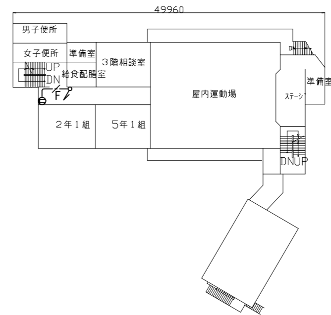
3階電源配線図 1:600
