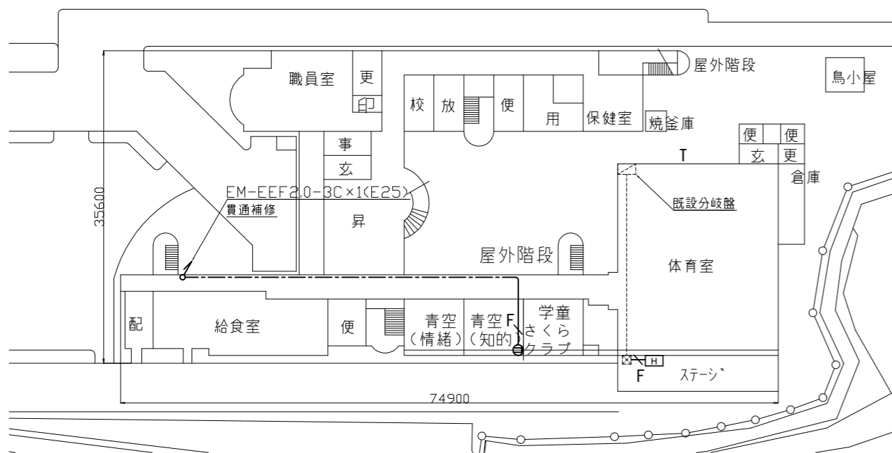
1階電源配線図 1:600
