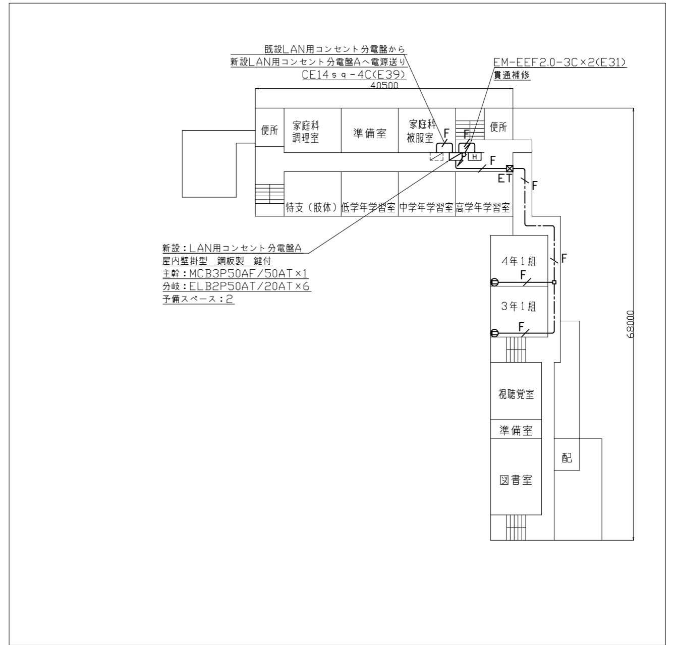
2階電源配線図 1:600
