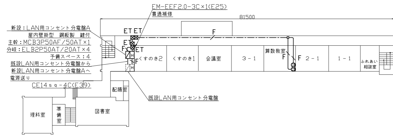
2階電源配線図 1:600
