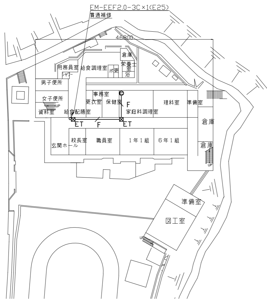
1階電源配線図 1:600
