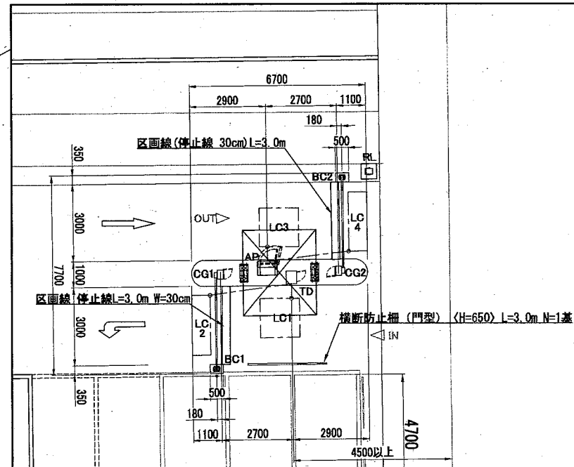
設置図 S=1/150 u:mm
