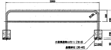
横断防止柵 S=1/40 u:mm
