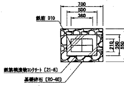
バーキャッチャー S=1/40 u:mm (2箇所)
