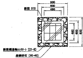
出庫警報灯 S=1/40 u:mm (1箇所)
