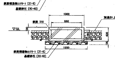
入口表示灯 S=1/40 u:mm (1箇所)
