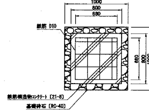
入口表示灯 S=1/40 u:mm (1箇所)
