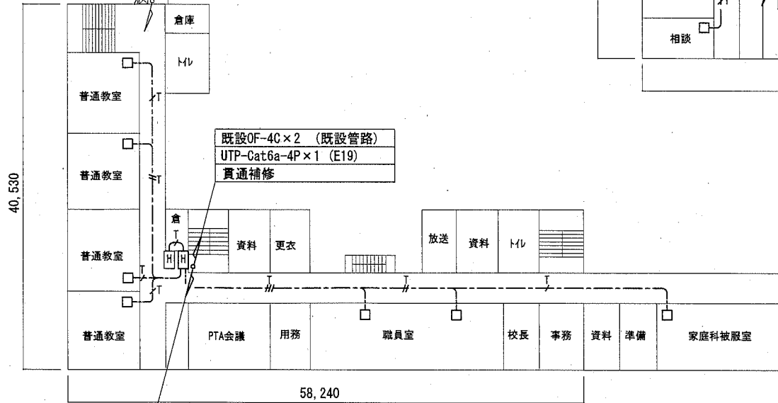
2階配線図 1/600
