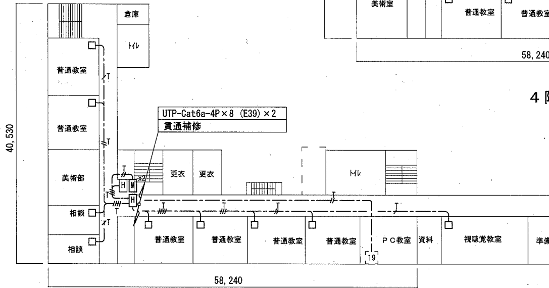
3階配線図 1/600
