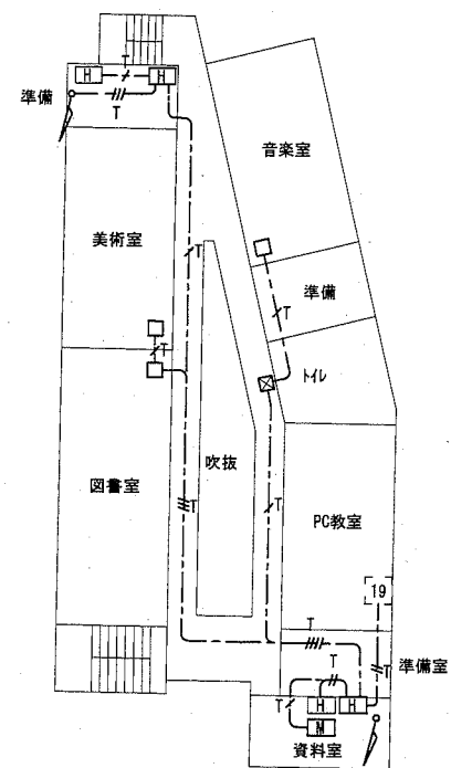
4階配線図 1/600
