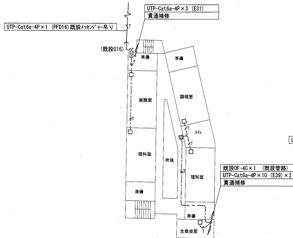
3階配線図 1/600
