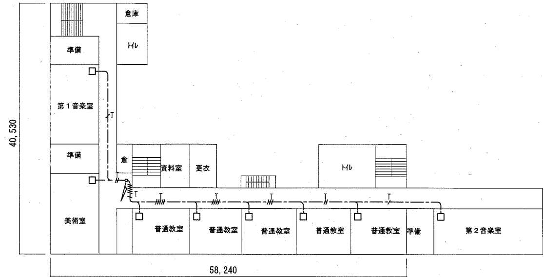
4階配線図 1/600
