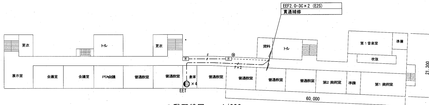
3階配線図 1/600
