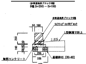
歩車道境界ブロック 1/30
