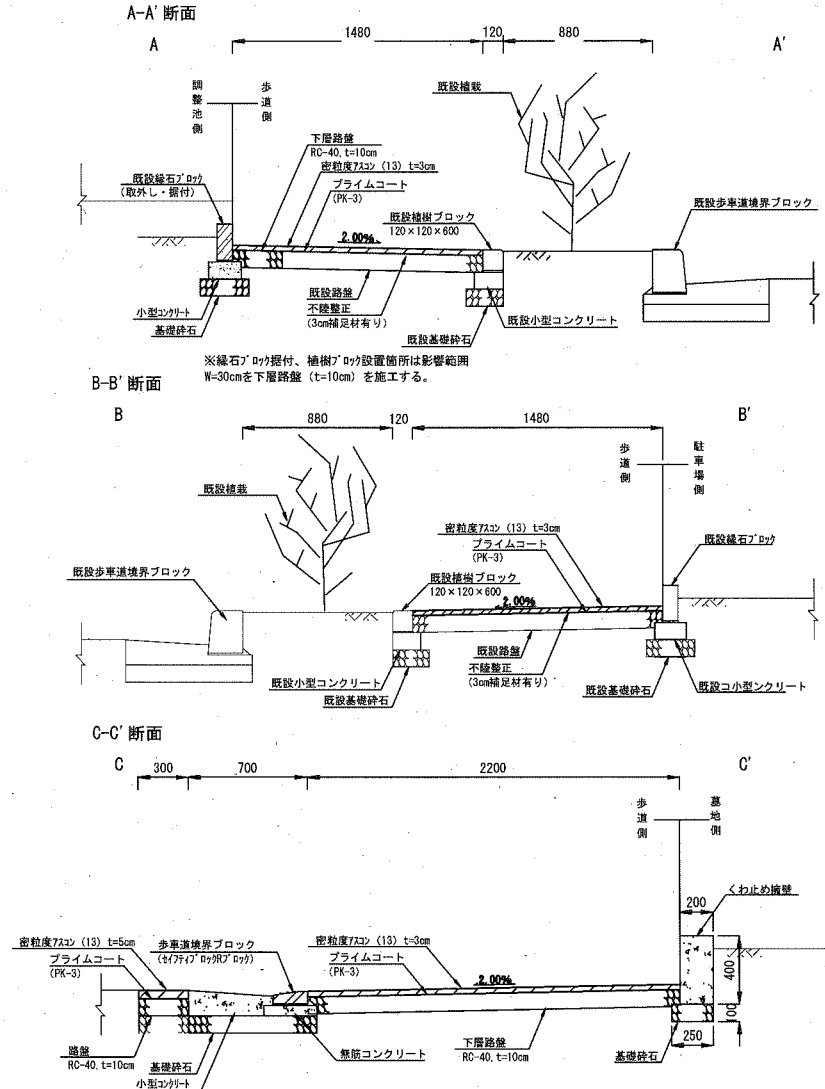
計画断面図
