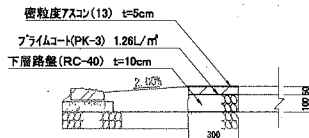
車道舗装 (切下げ部) 1/30
