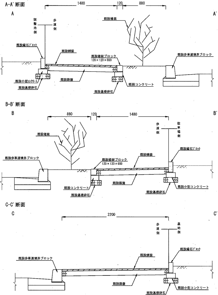
現況断面図
