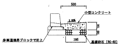
L型側溝 1/30
