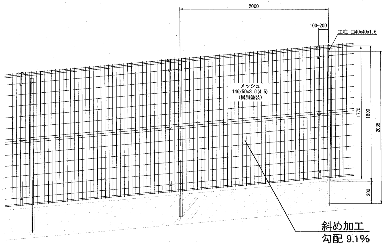
立入防止柵構造図 S=1:30
