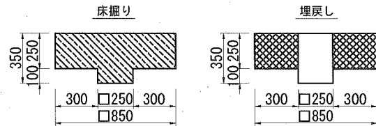
断面図
