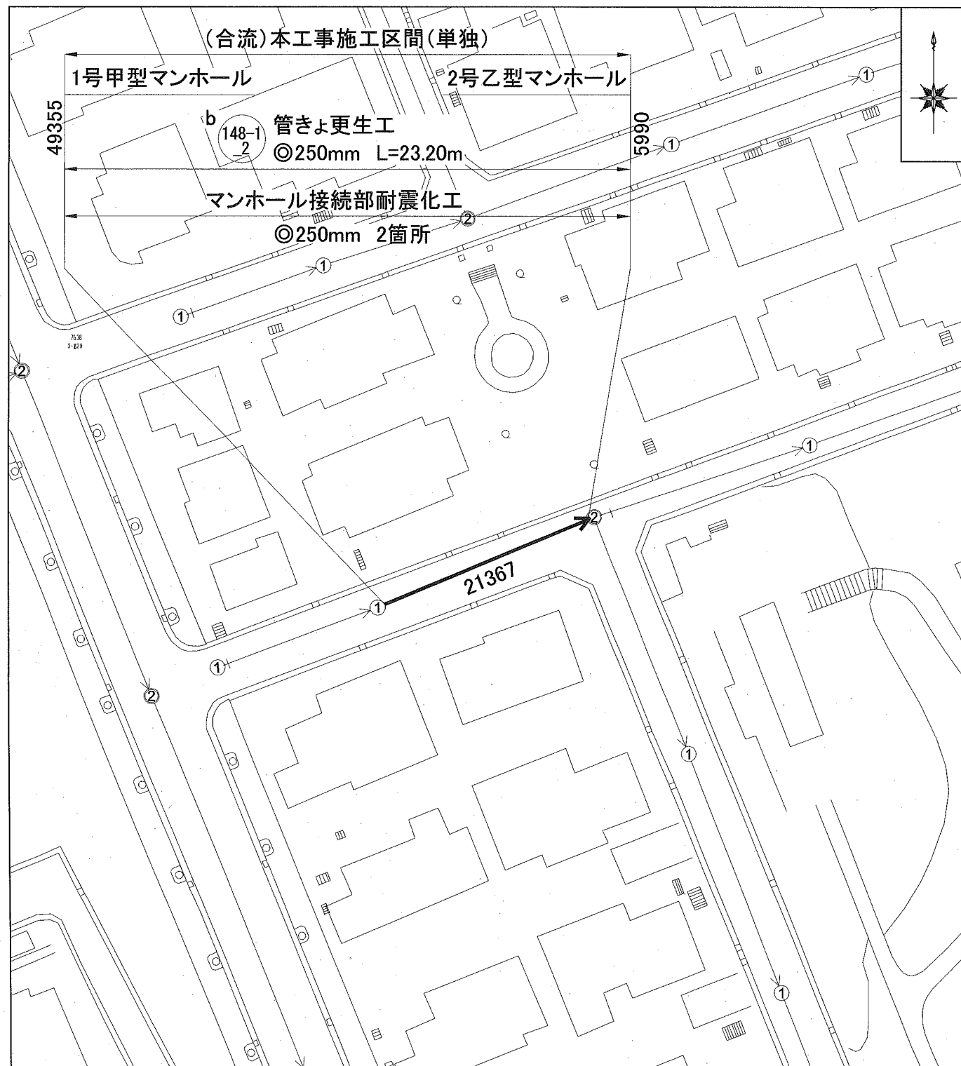
平面図(2/3) S=1:500
