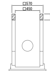
雨水樹 [Φ450]
