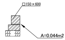
地先境界ﾌﾞﾛｯｸ 10m当り
