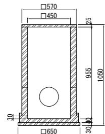
汚水樹 [φ450] 1基当り
