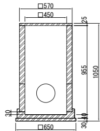
汚水樹 [Φ450]
