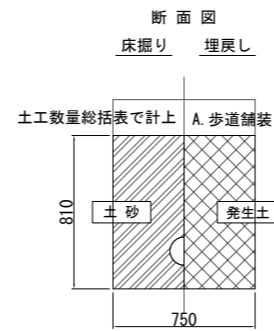
硬質塩化ビニル管 [Φ150]
