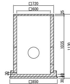
汚水樹 [Φ600]①
