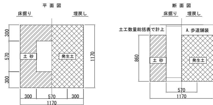
汚水樹 [Φ450]
