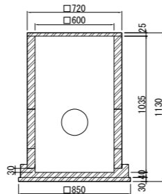
汚水樹 [φ600]①
