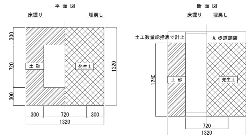
汚水樹 [Φ600]②
