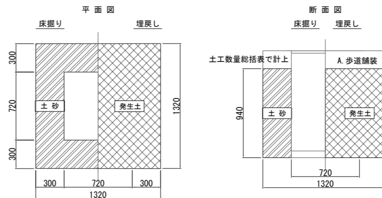
汚水樹 [Φ600]①
