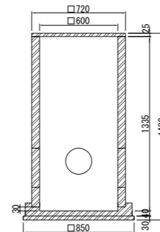
汚水樹 [φ600]② 1基当り
