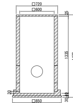
汚水樹 [Φ600]②
