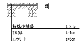
土間ｺﾝｸﾘｰﾄ 10m2当り
