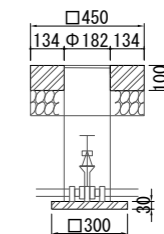
仕切弁きょう
