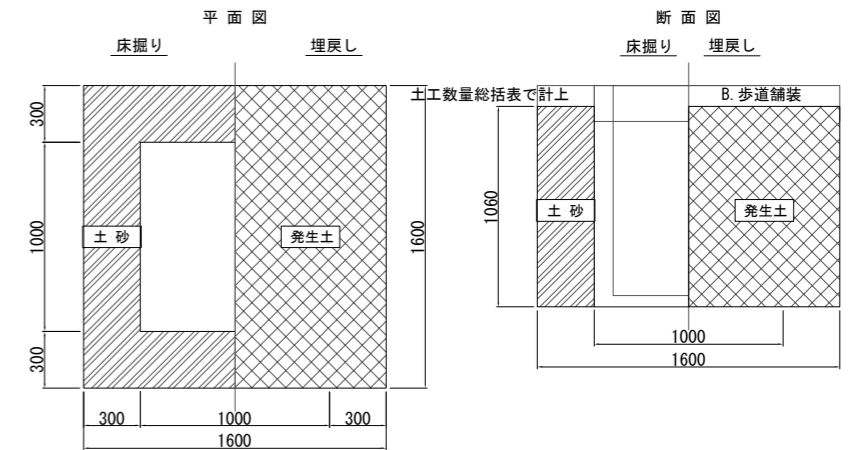
電気用ハンドホール
