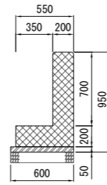
断面図
