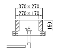
散水栓
