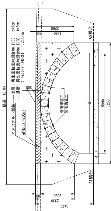
平面図
