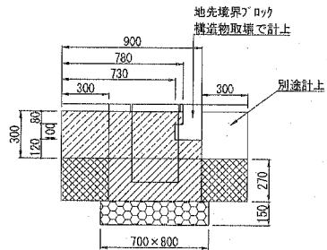
A. 雨水ます部分 L=1.3m (余掘含む) 【A-A断面】
