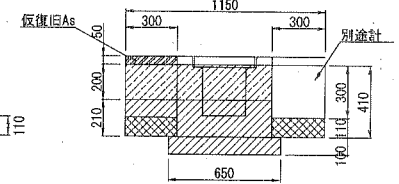
横断水抜き③部分 施工延長 L=4.4m 【B-B断面】
