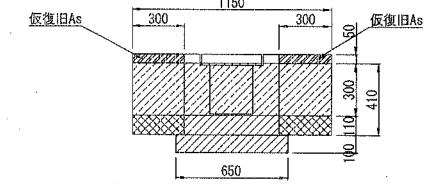
横断水抜き①部分 施工延長 L=2.9m 【B-B断面】
