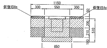
横断水抜き④部分 施工延長 L=3.0m 【A-A断面】
