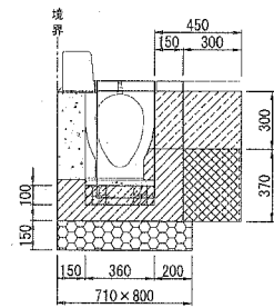
C. 雨水ます部分 L=0.7m 【C-C断面】
