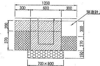
A. 雨水ます部分 L=2.6m (余掘含む) 【A-A断面, C-C断面】
