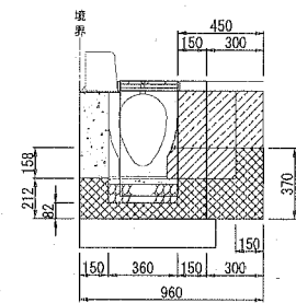
余掘部分 L=0.6m 【B-B, D-D断面】
