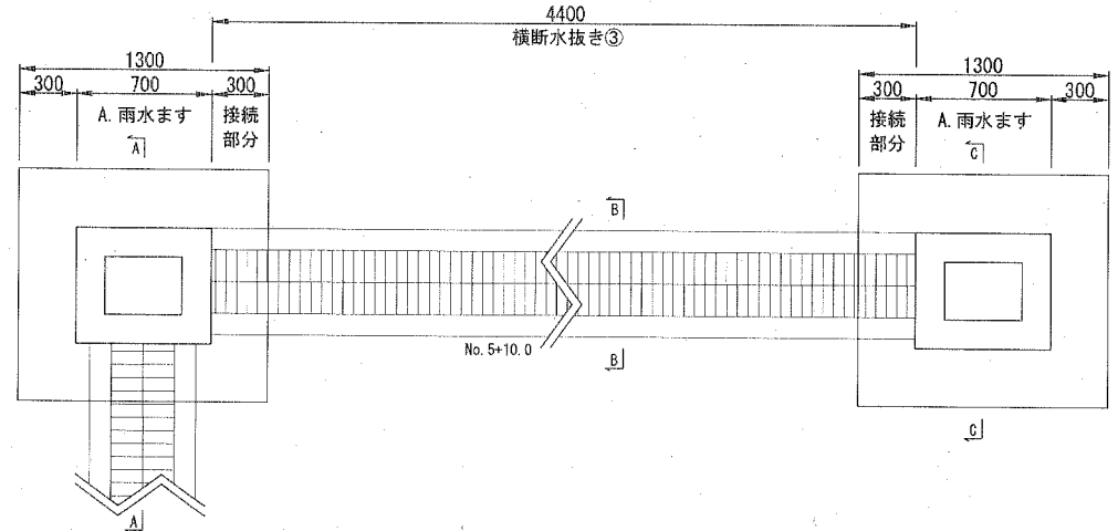
A. 雨水ます部分 L=2.6m (余掘含む) 【A-A断面, C-C断面】
