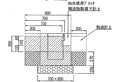
A. 雨水ます部分 L=1.3m(余掘含む) 【A-A断面】
