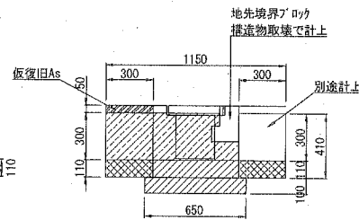
横断水抜き②部分 施工延長 L=7.2m 【B-B断面】
