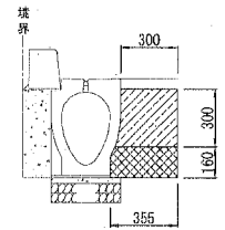
プラスチック側溝部分 L=2.7m 【A-A断面, E-E断面】
