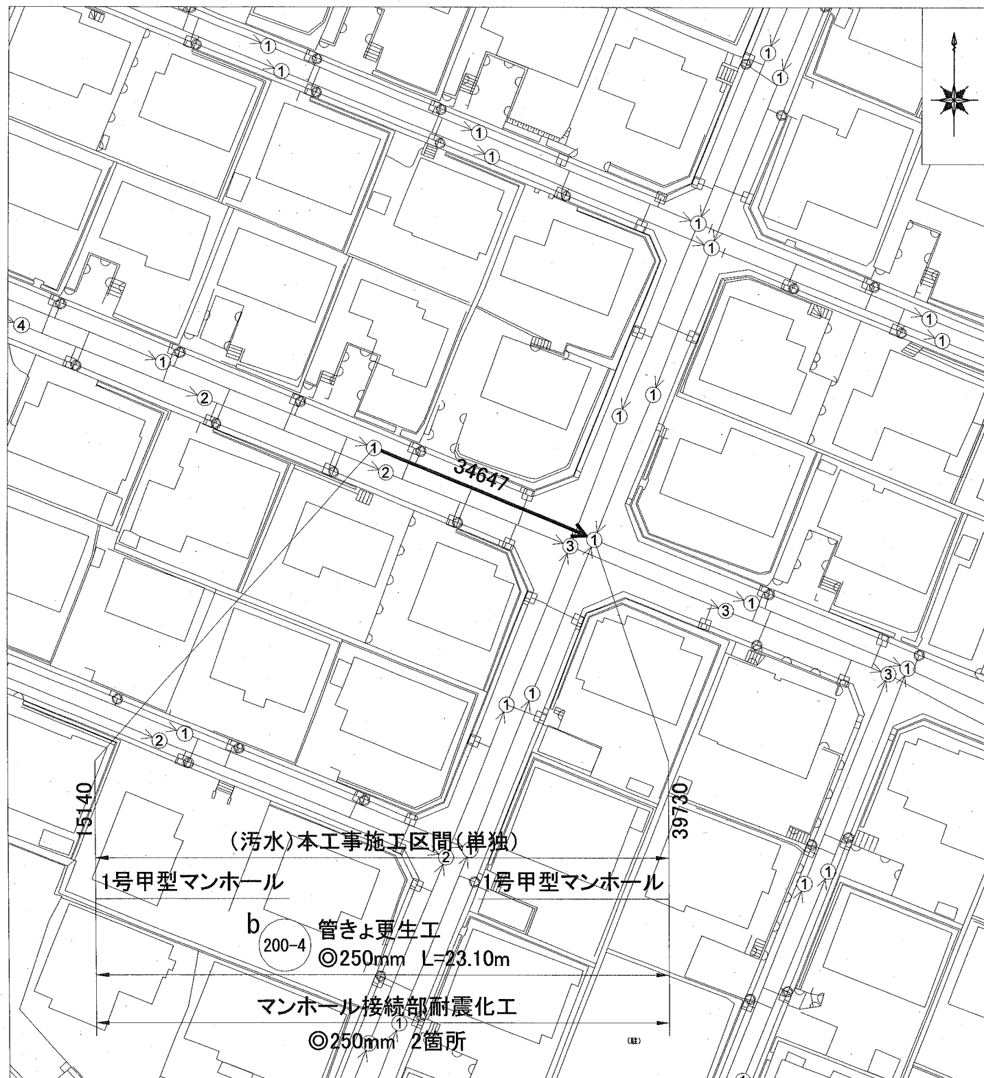
平面図 (2/3) S=1:500
