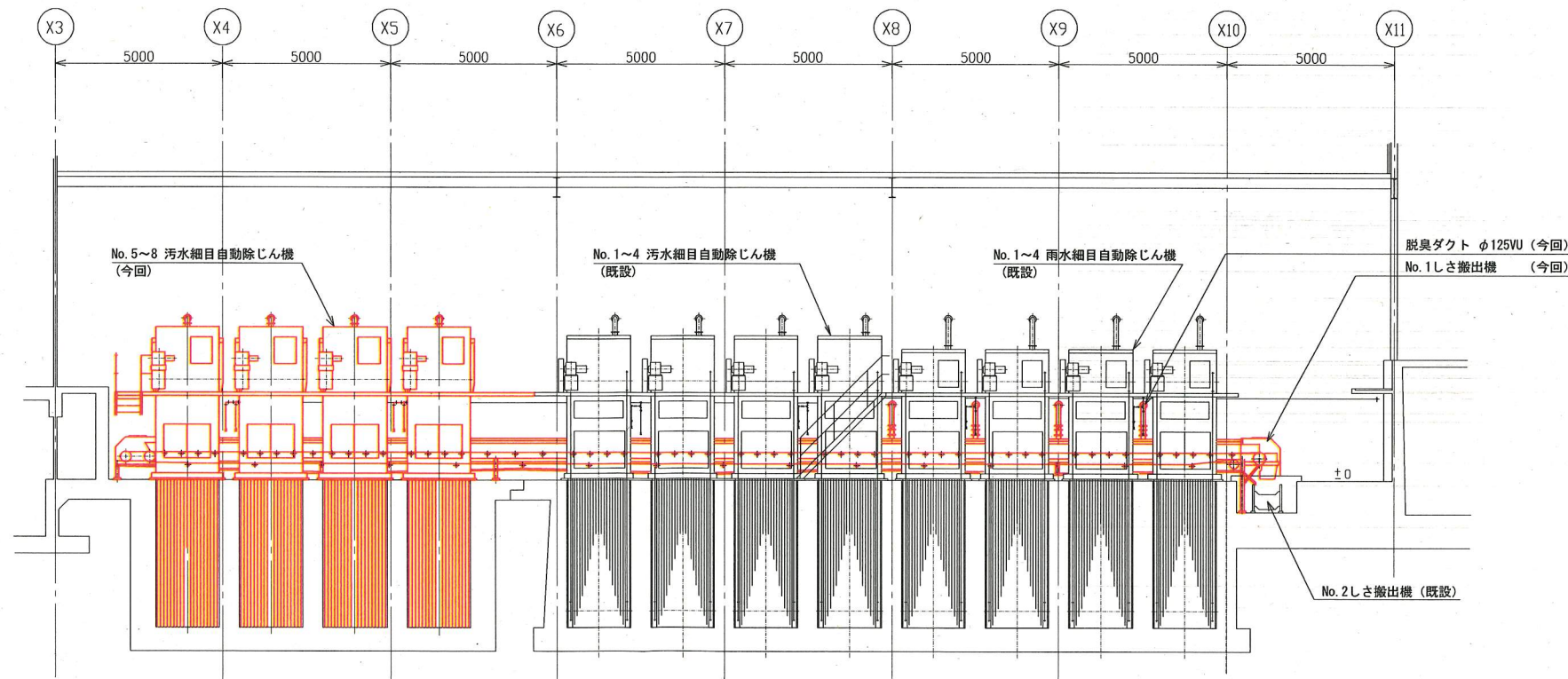
B-B 断面図 (S=1/100)
