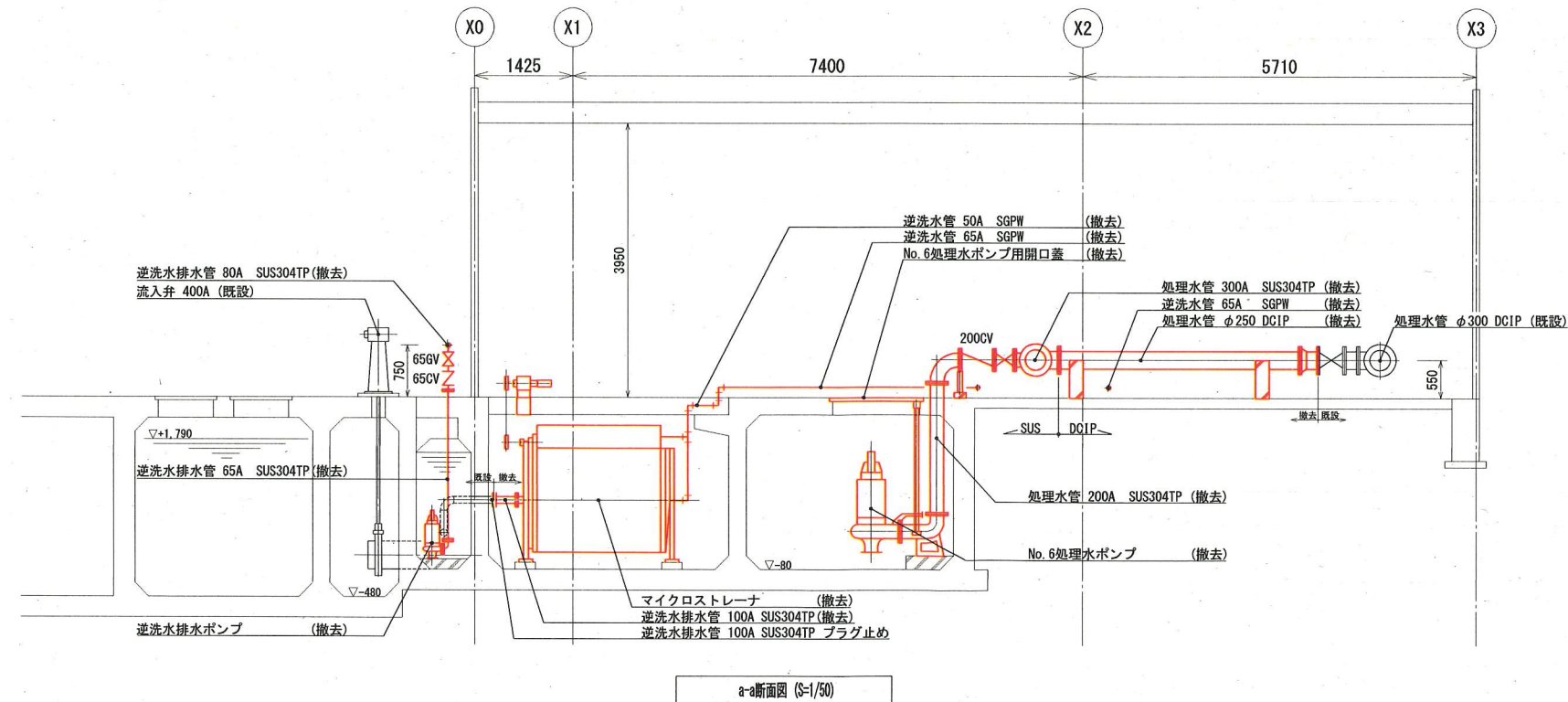
処理水ポンプ室撤去平面図 (S=1/50)
