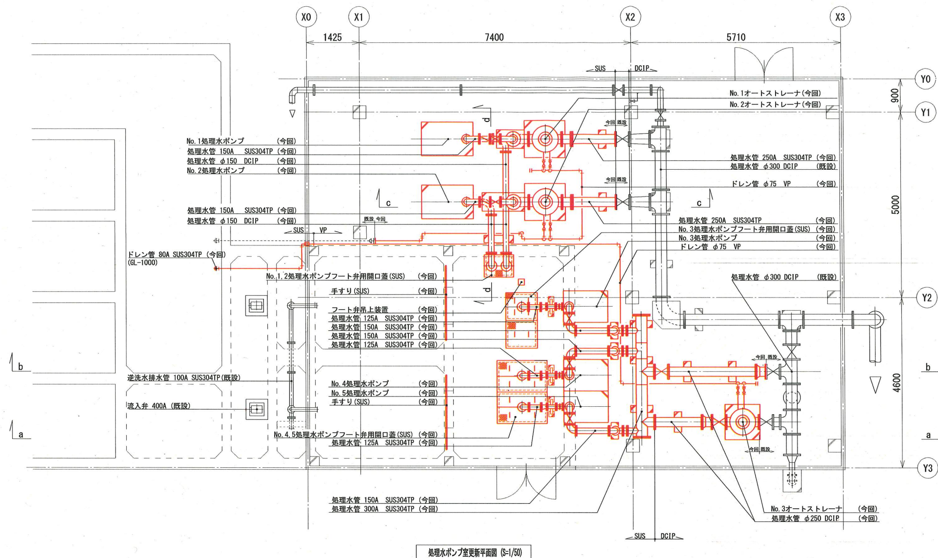
処理水ポンプ室更新平面図 (S-1/50)
