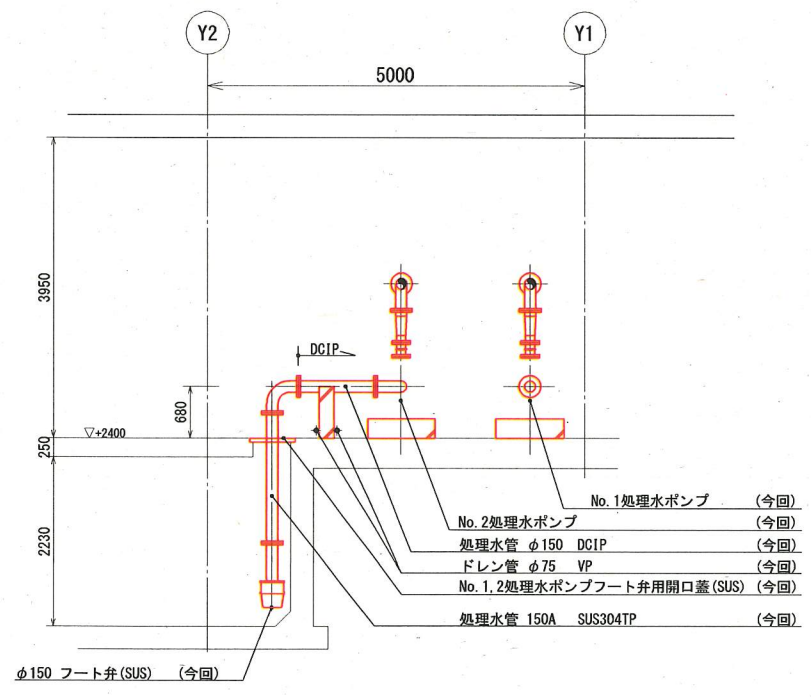
d-d断面図 (S=1/50)
