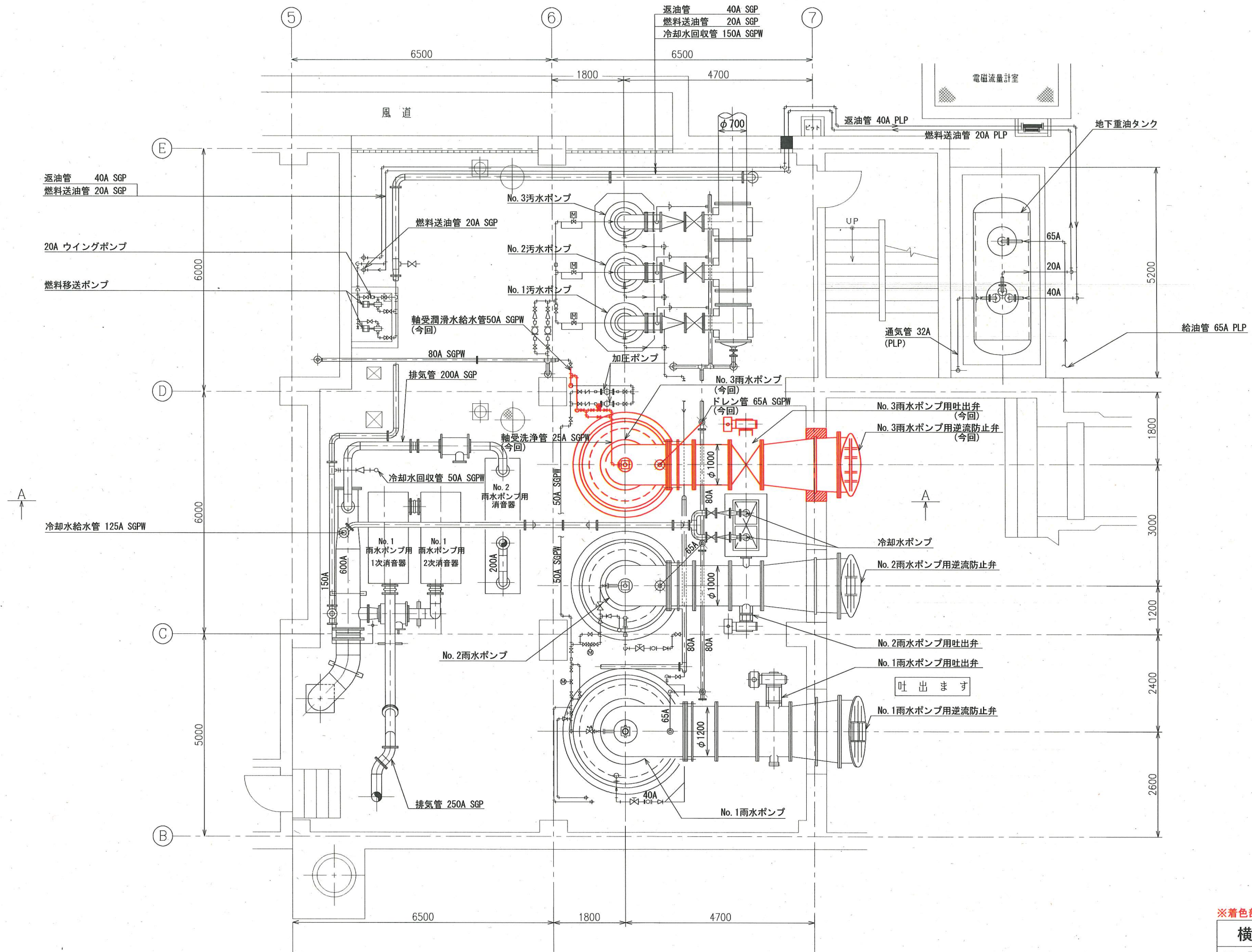
地下1階平面図 (S=1/50)
