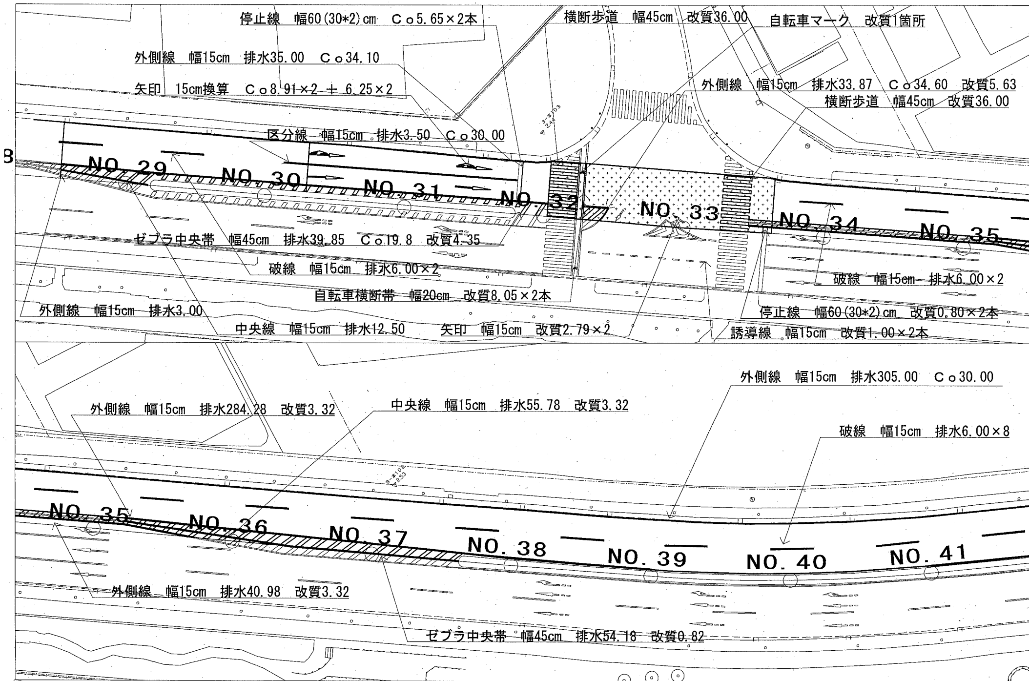
別図-3 (non scale)
