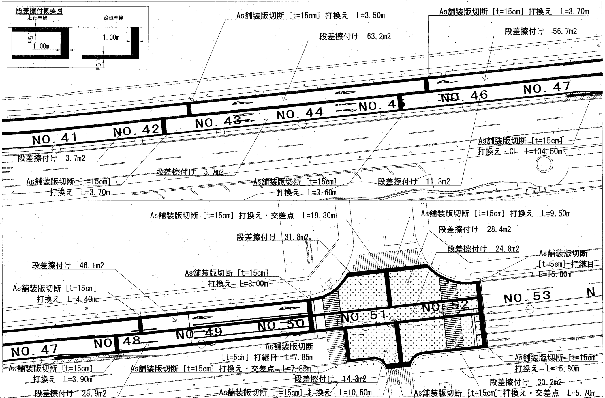
別図-2 (non scale)
