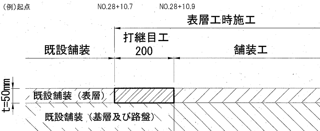
打継目工概略図
