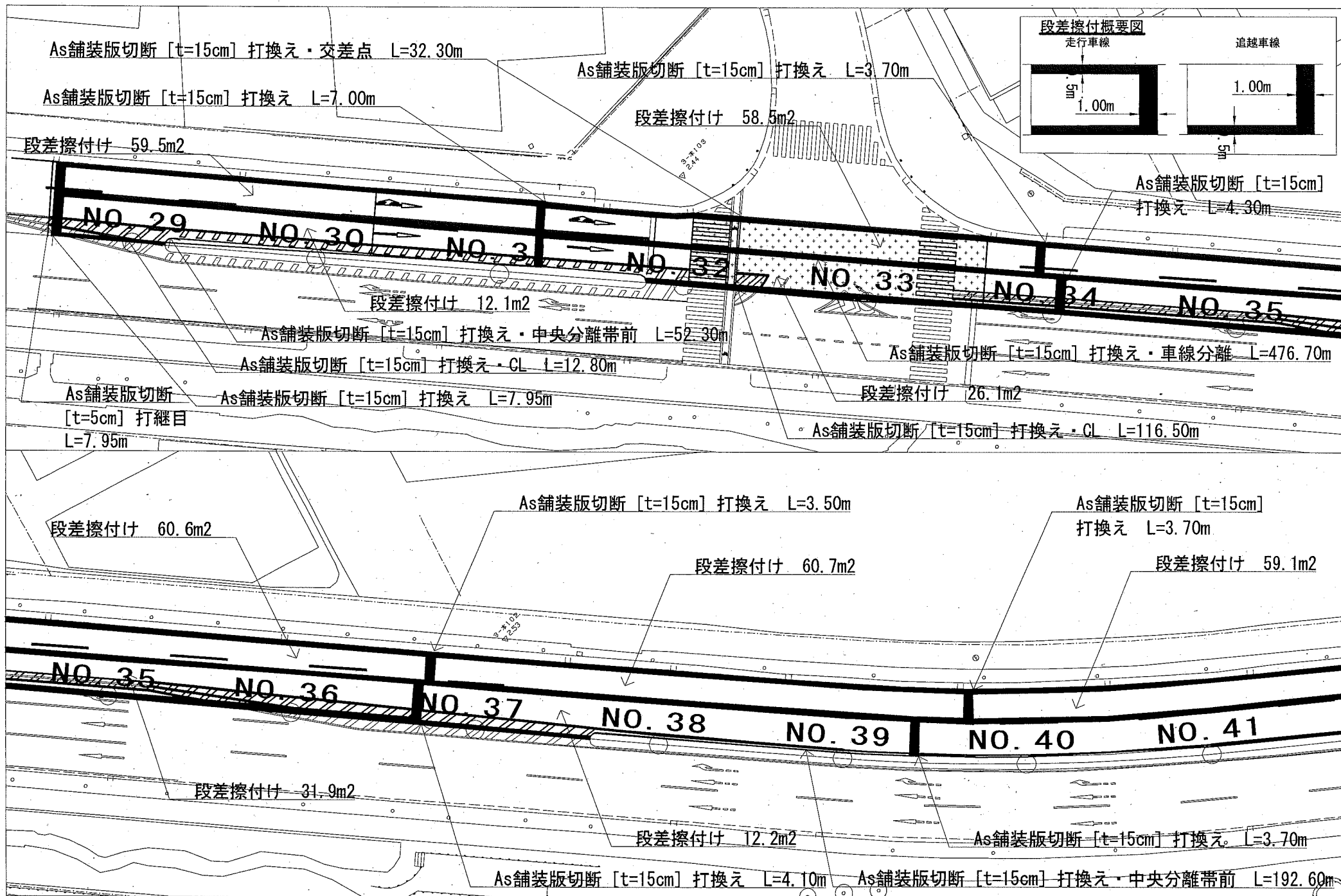
別図-1 (non scale)
