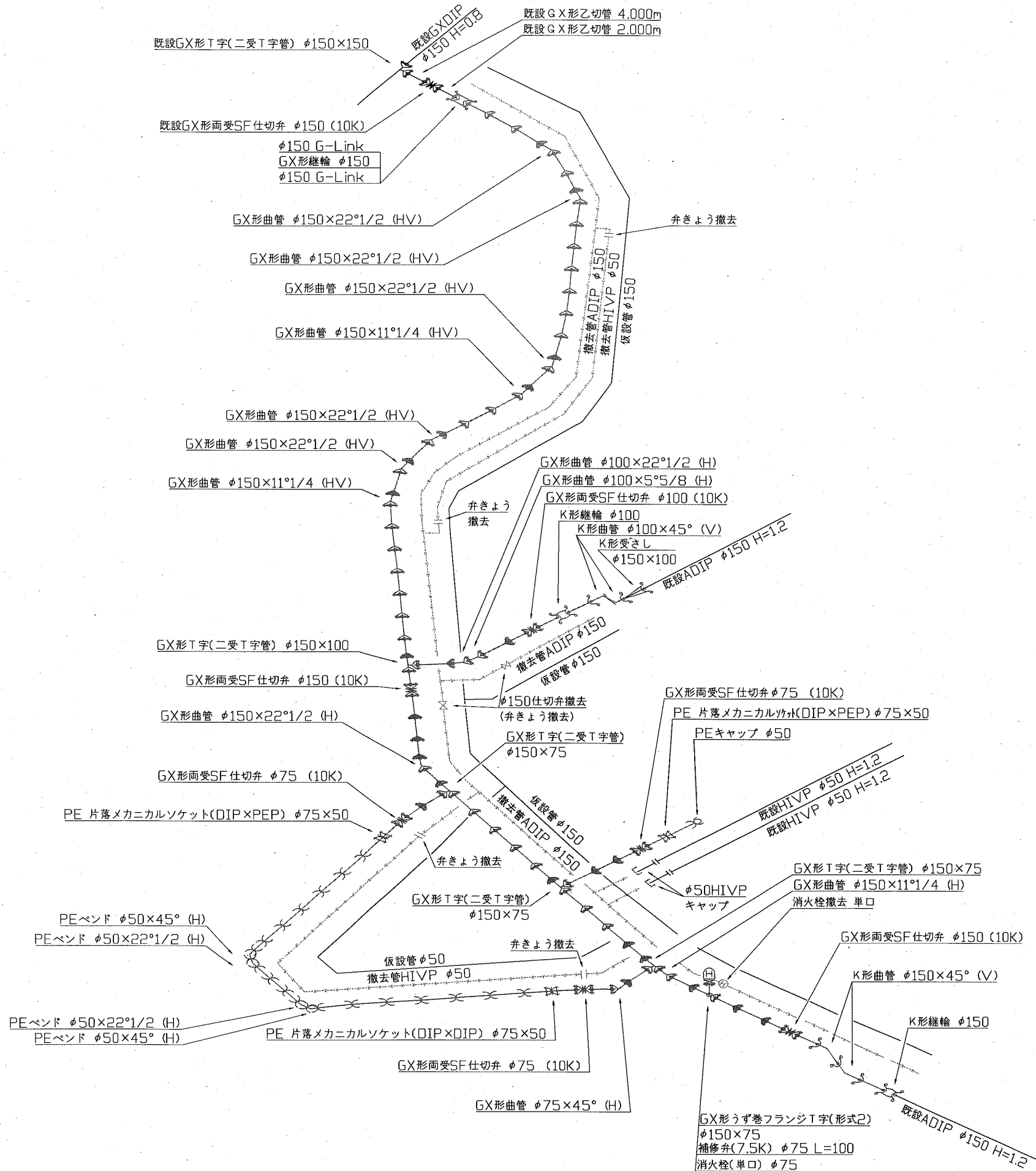
配管図
