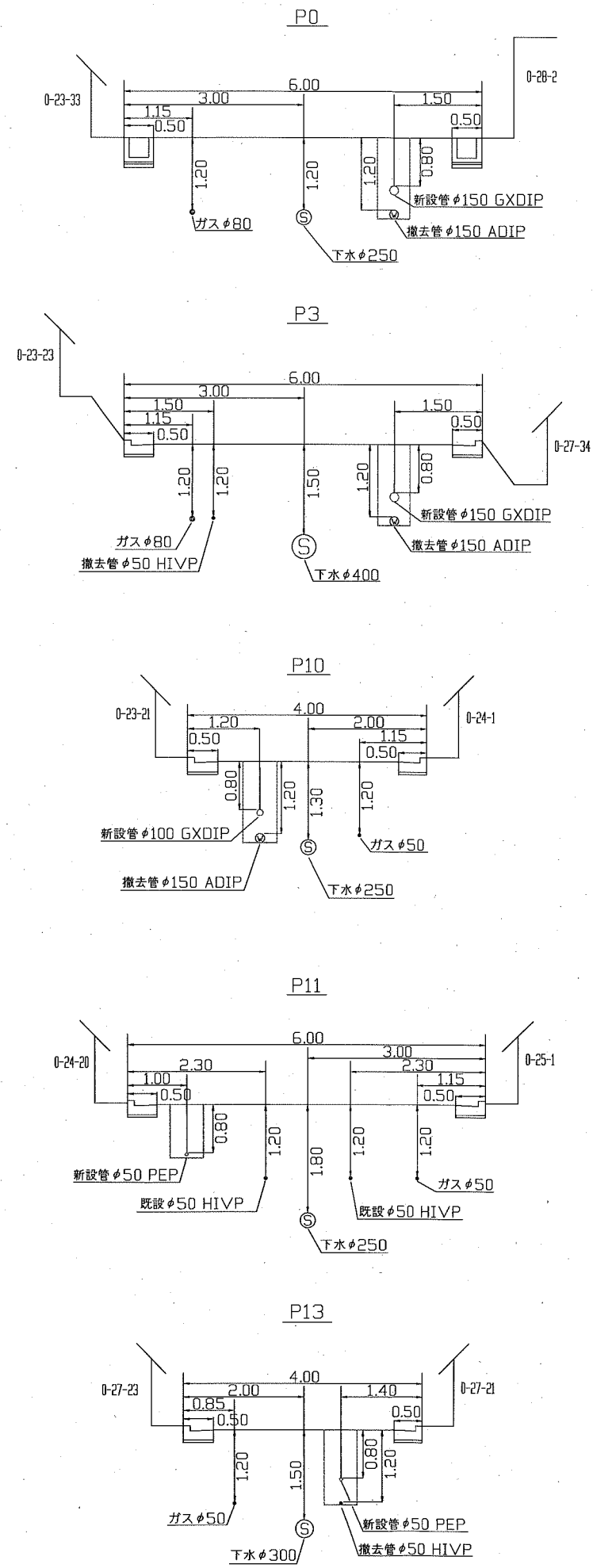
断面図 S=1/50
