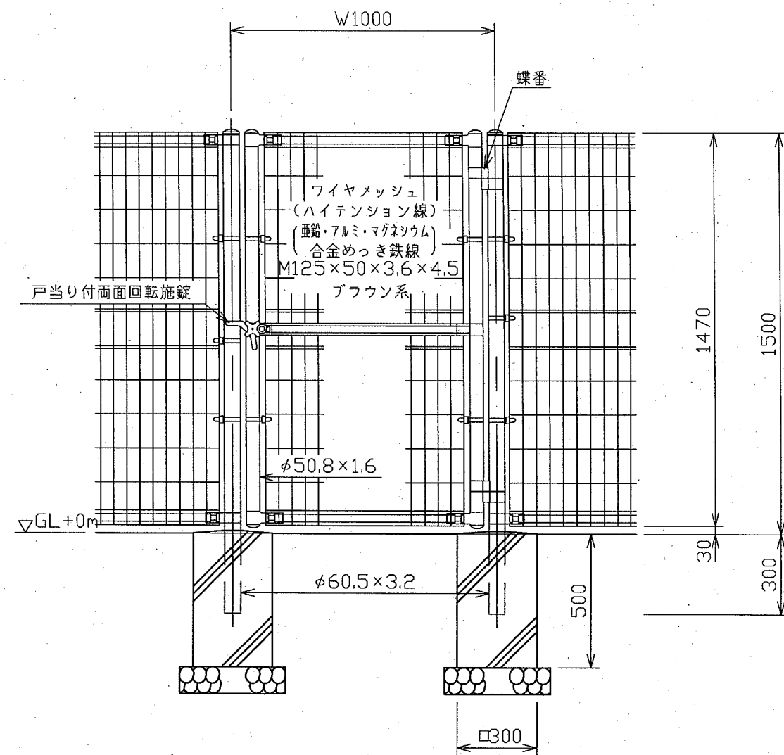
門柱・扉枠位置関係図 S=1/5
