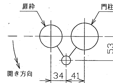
門柱・扉枠位置関係図 S=1/5
