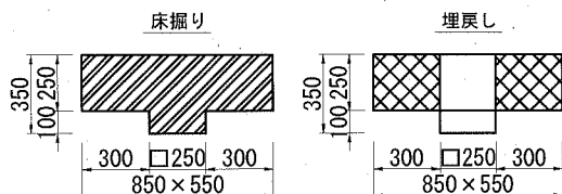
断面図
