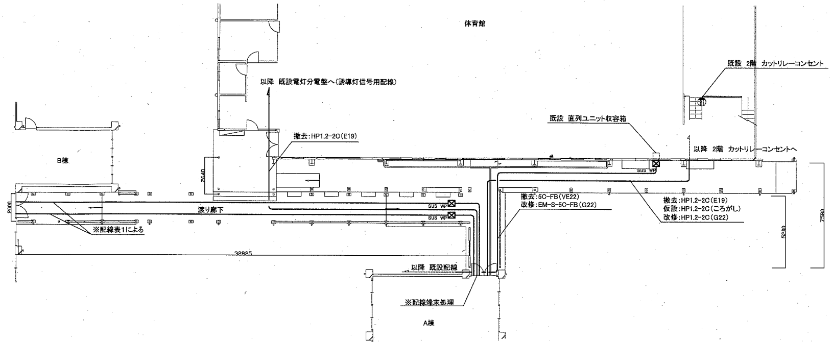
渡り廊下 弱電設備 改修図 1:200
