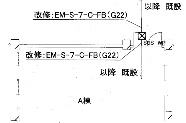
A棟 外壁 改修図 1:100
