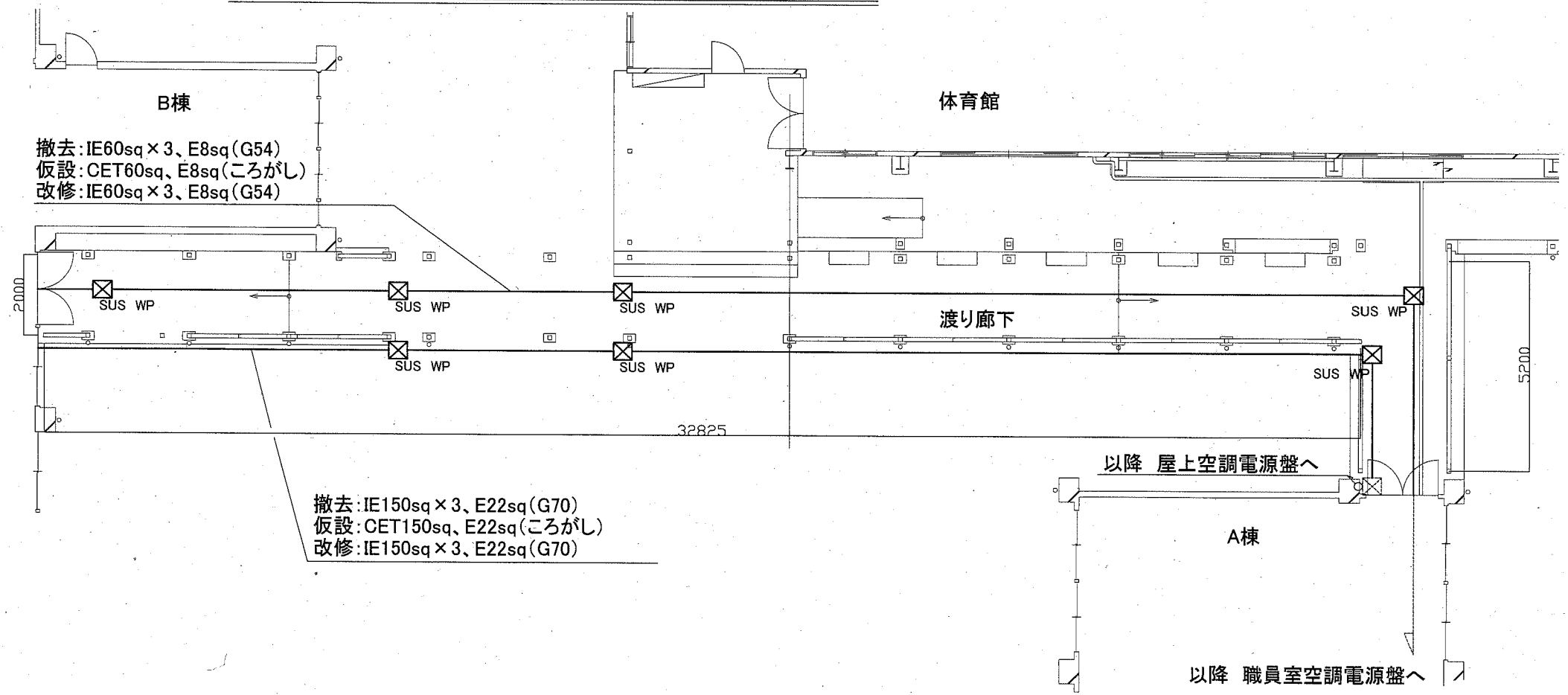
渡り廊下 電灯設備 改修図 1:200
