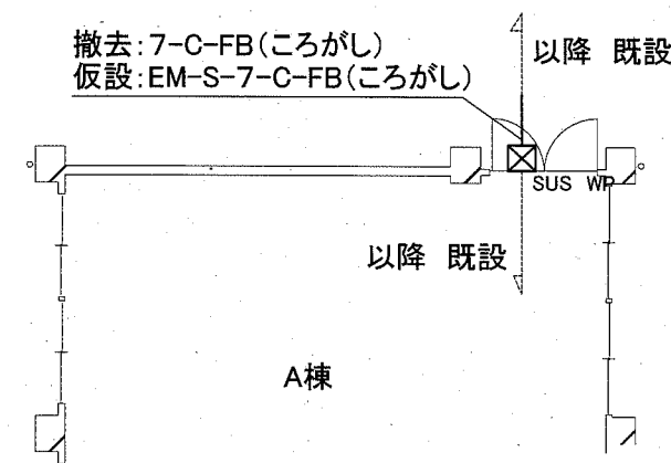
A棟 外壁 撤去図 1:100
