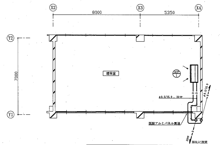
1階改修平面図 1:100
