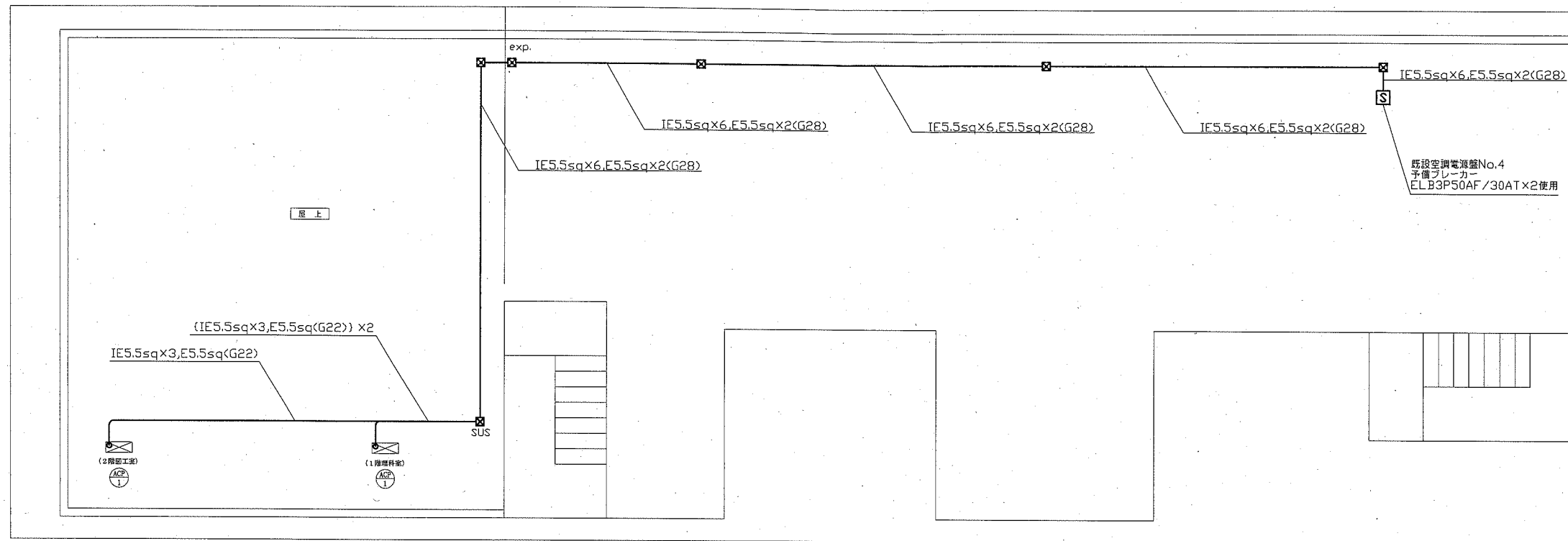
衣笠小学校電気改修図 1:100
