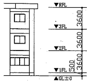
階高図 N.S.
