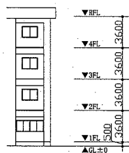
C棟階高図 N.S.
