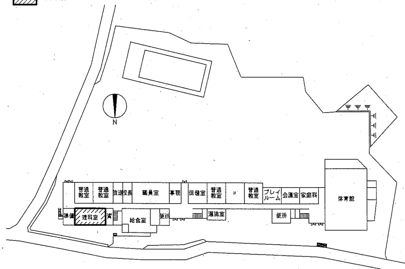
配置図兼1階平面図 1:800
