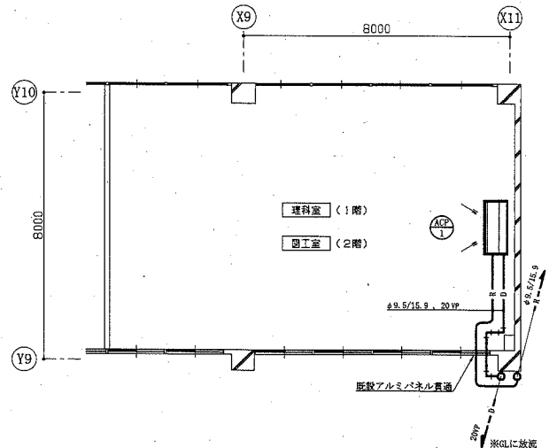
C棟1階・2階改修平面図 1:100
