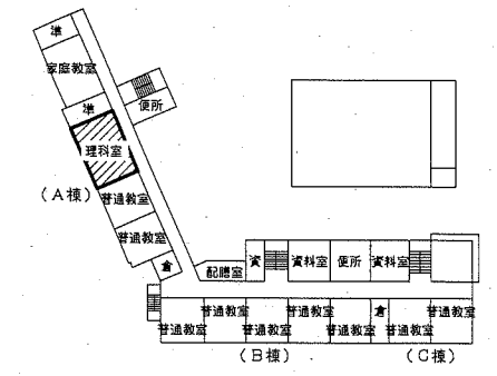
2階平面図 1:800
