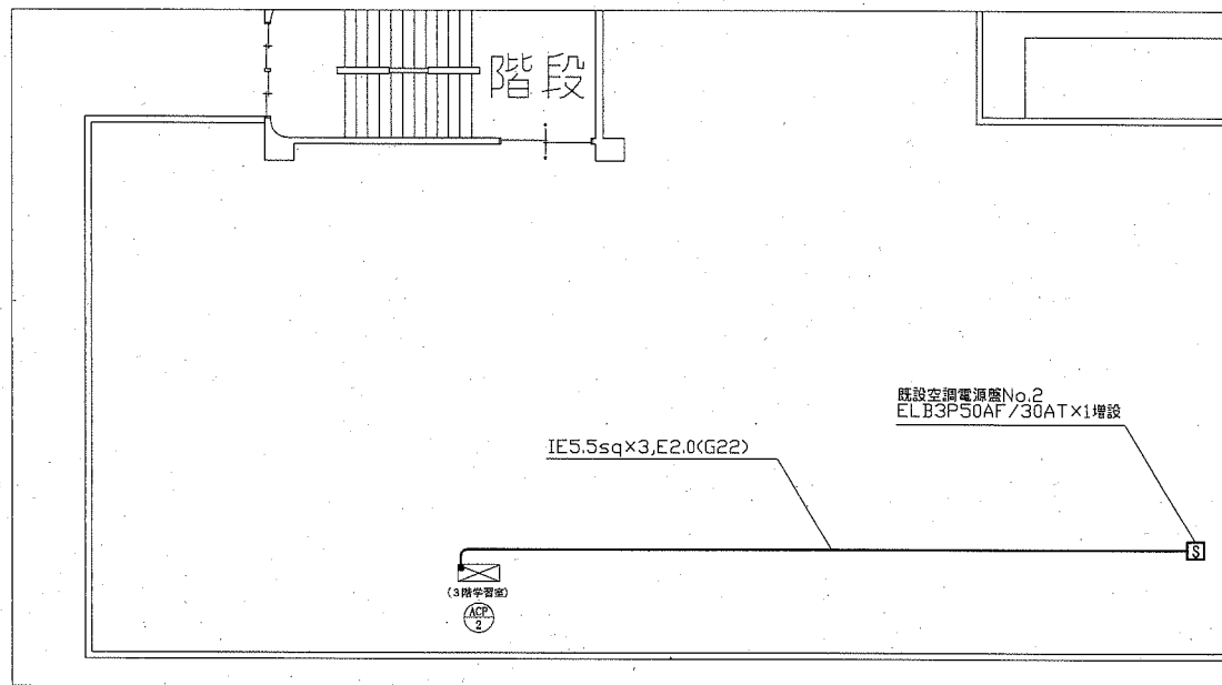
森崎小学校B棟電気改修図 1:100
