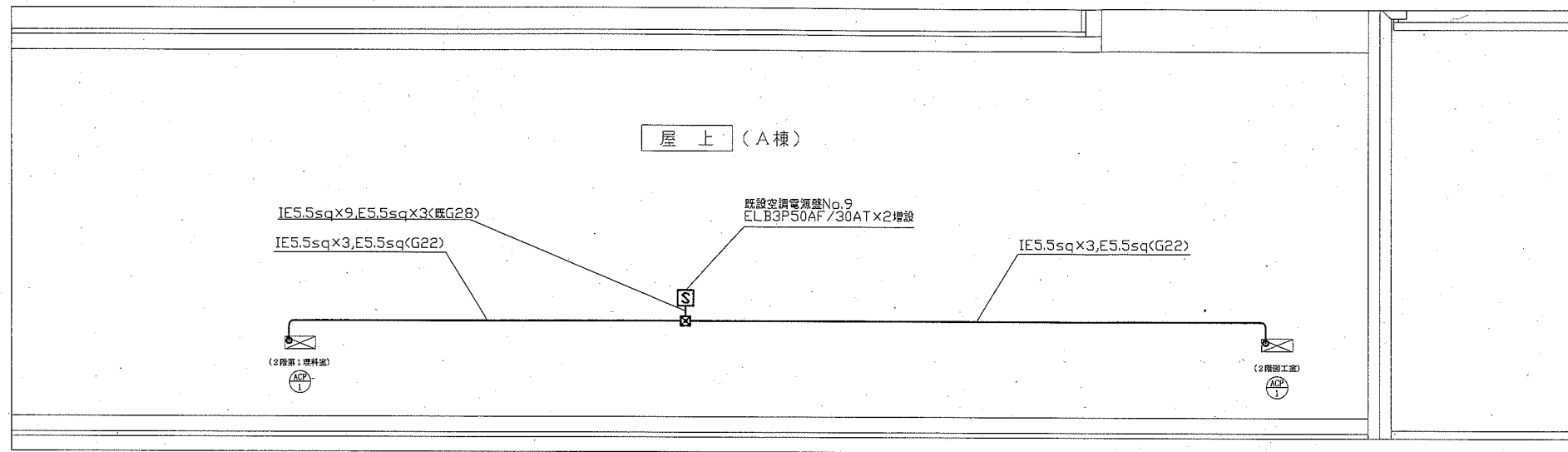
森崎小学校A棟電気改修図 1:100
