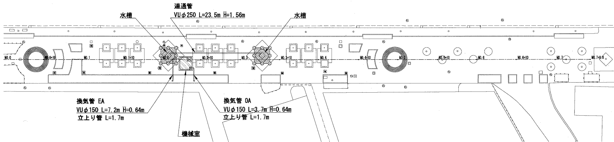
機械室 S=1/100
