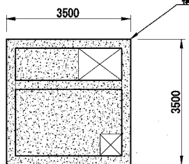
平面図 (下部)
