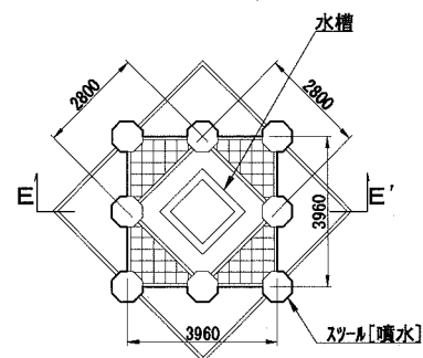
平面図 S=1/150
