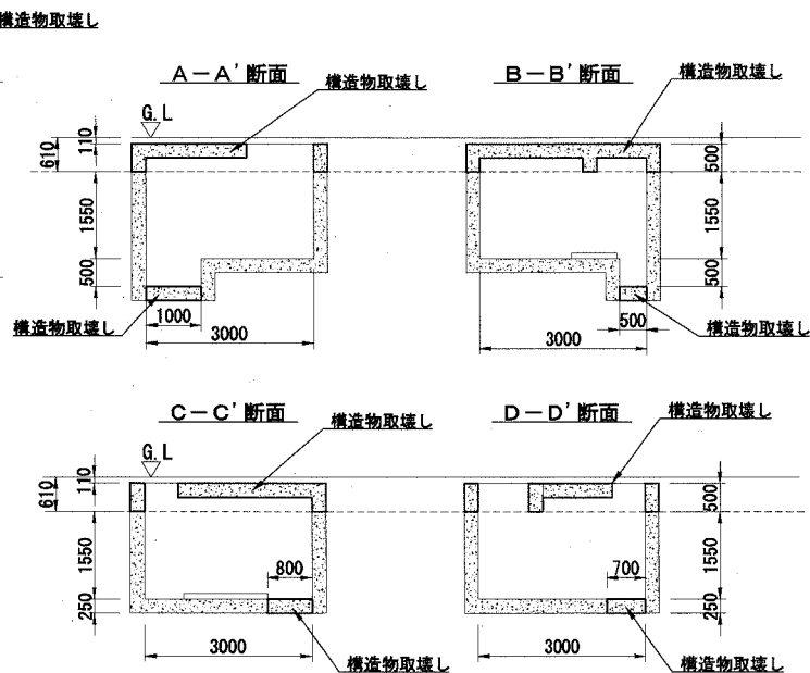
機械室 S=1/100
