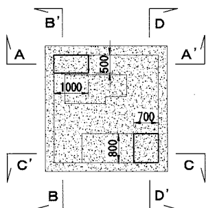
平面図 (下部)
