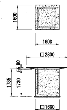
水槽 S=1/100
