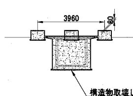
E-E' 断面
