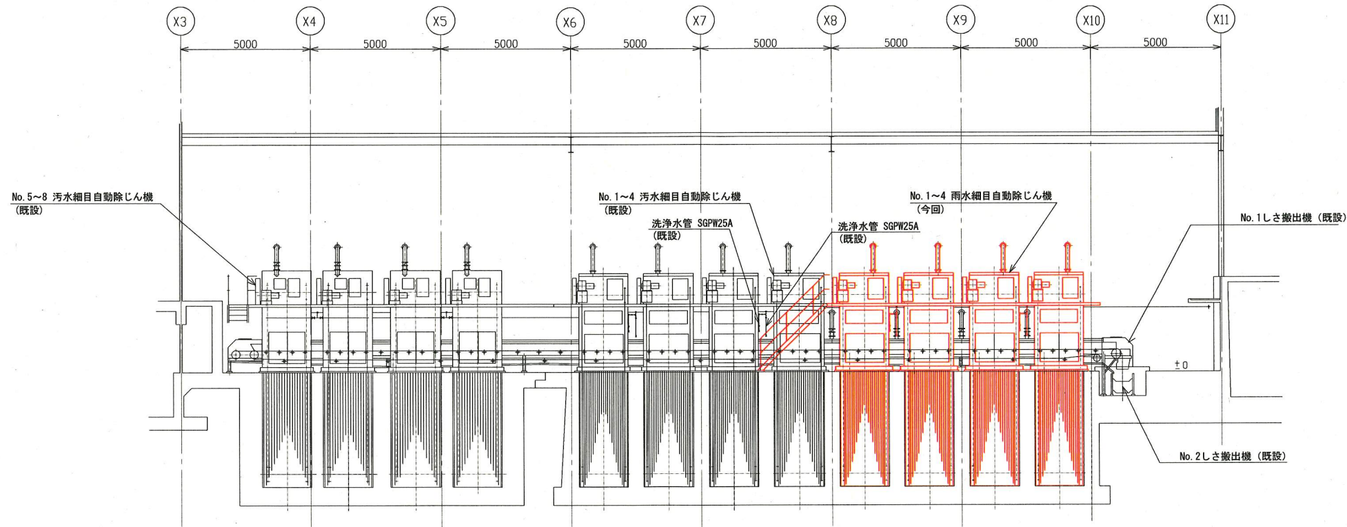
B-B 断面図 (S=1/100)
