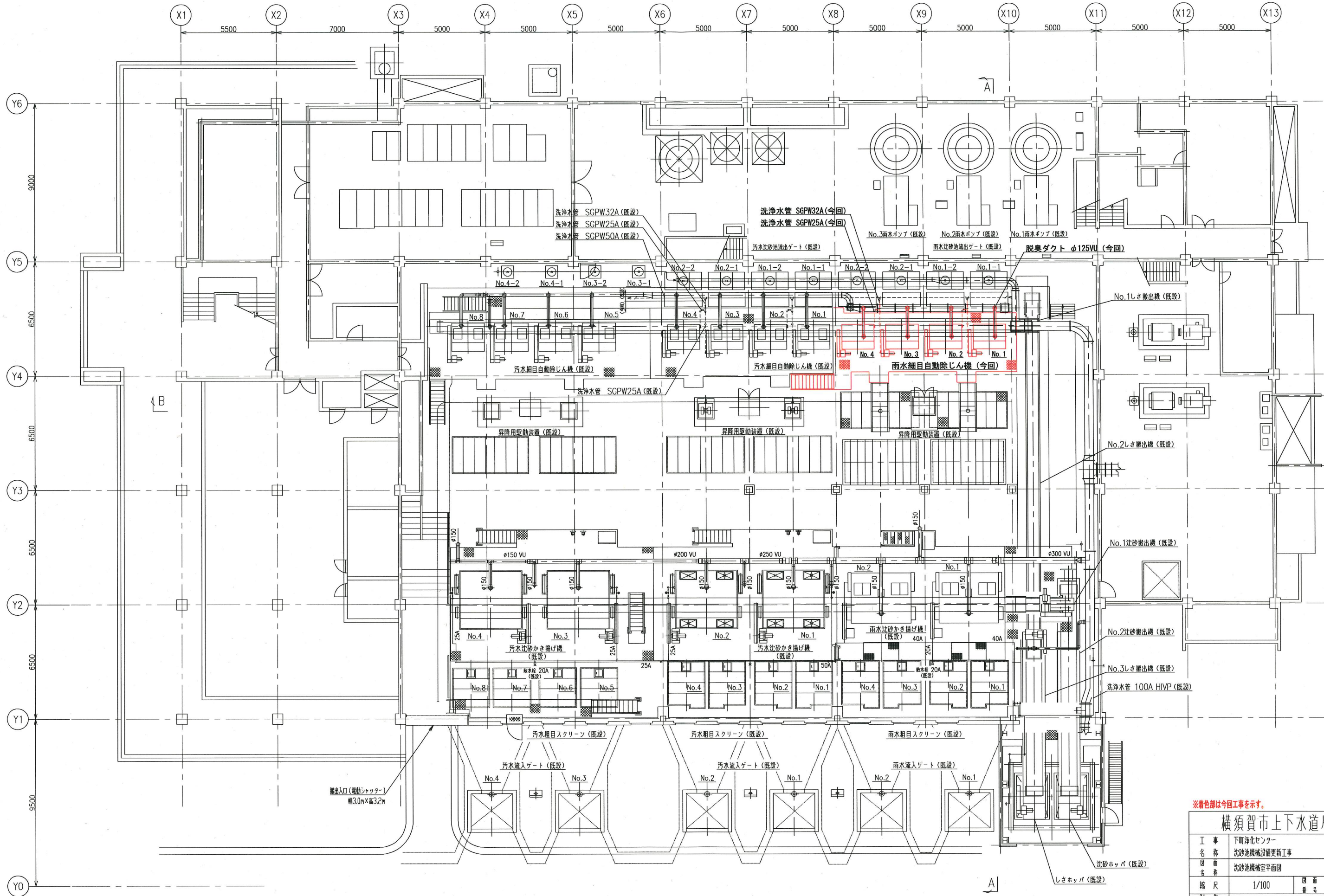
沈砂池機械室平面図 (S=1/100)
