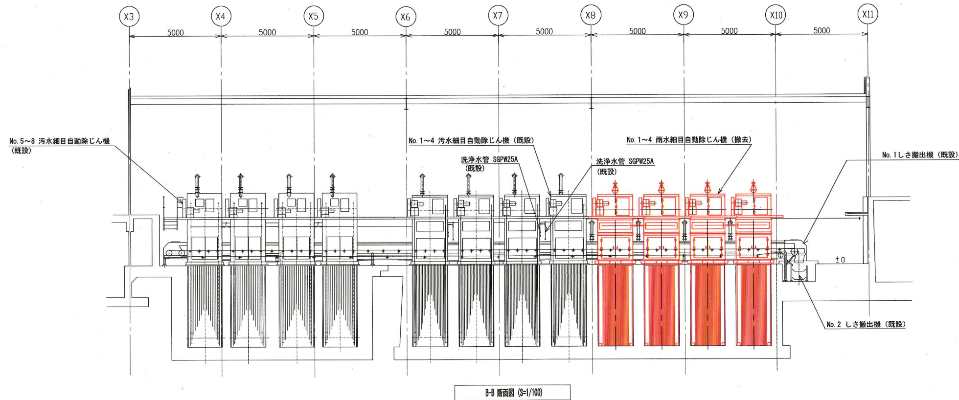
B-B 断面図 (S=1/100)
