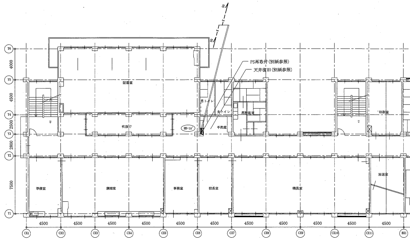
2階配管平面図(新設) 1:200
