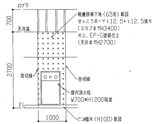
3階PS壁新設詳細図 1/50
