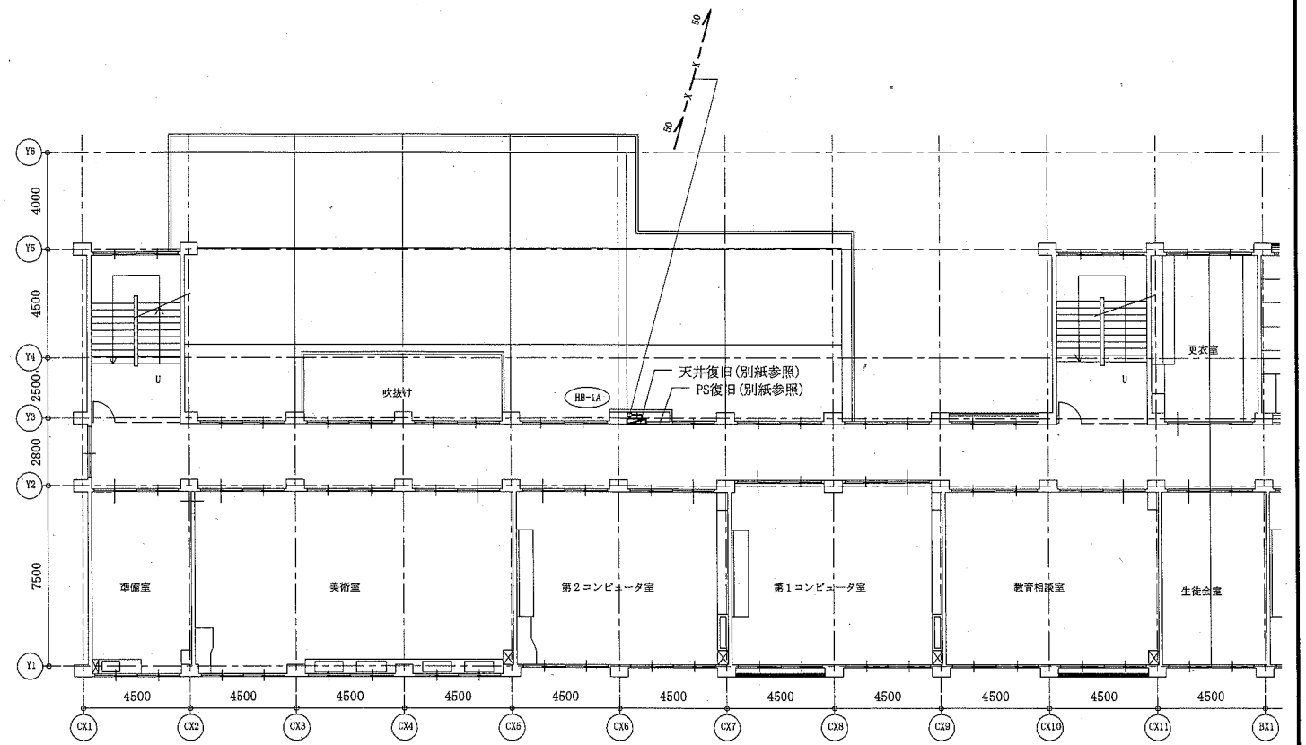
3階配管平面図(新設) 1:200
