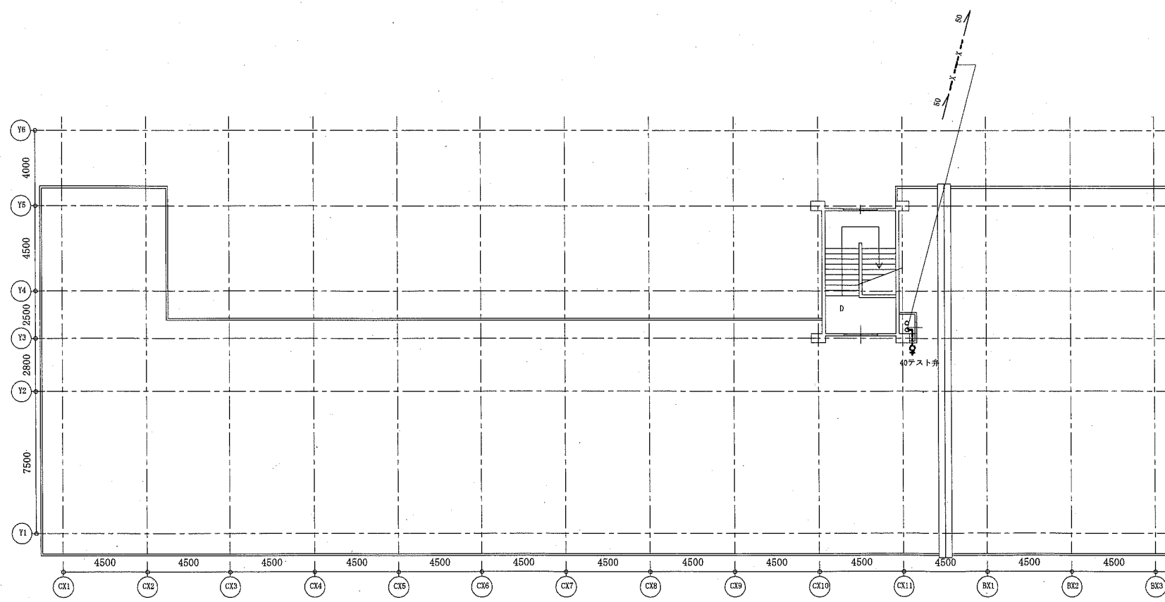
屋上階配管平面図(撤去) 1:200
