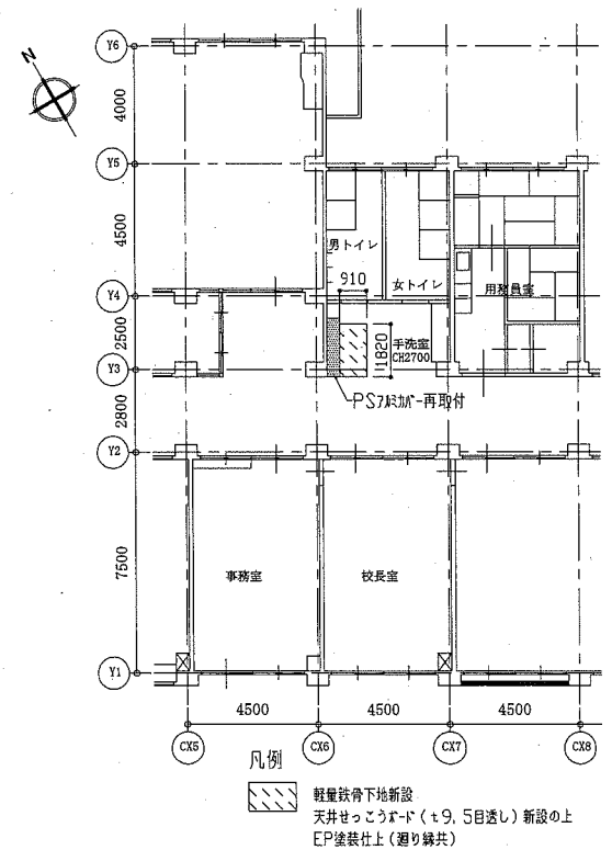
2階天井伏図 1/200
