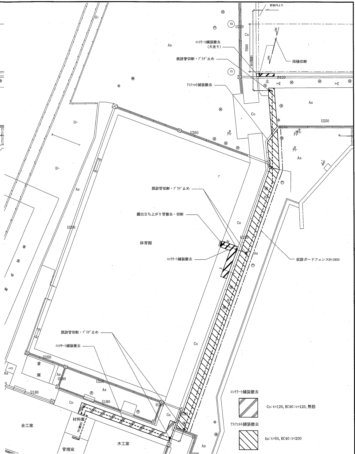
外構配管平面図(撤去) 1:200 ※撤去以外の土中既設管は残置とする (機械設備)
