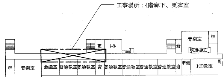
4階平面図 1:800
