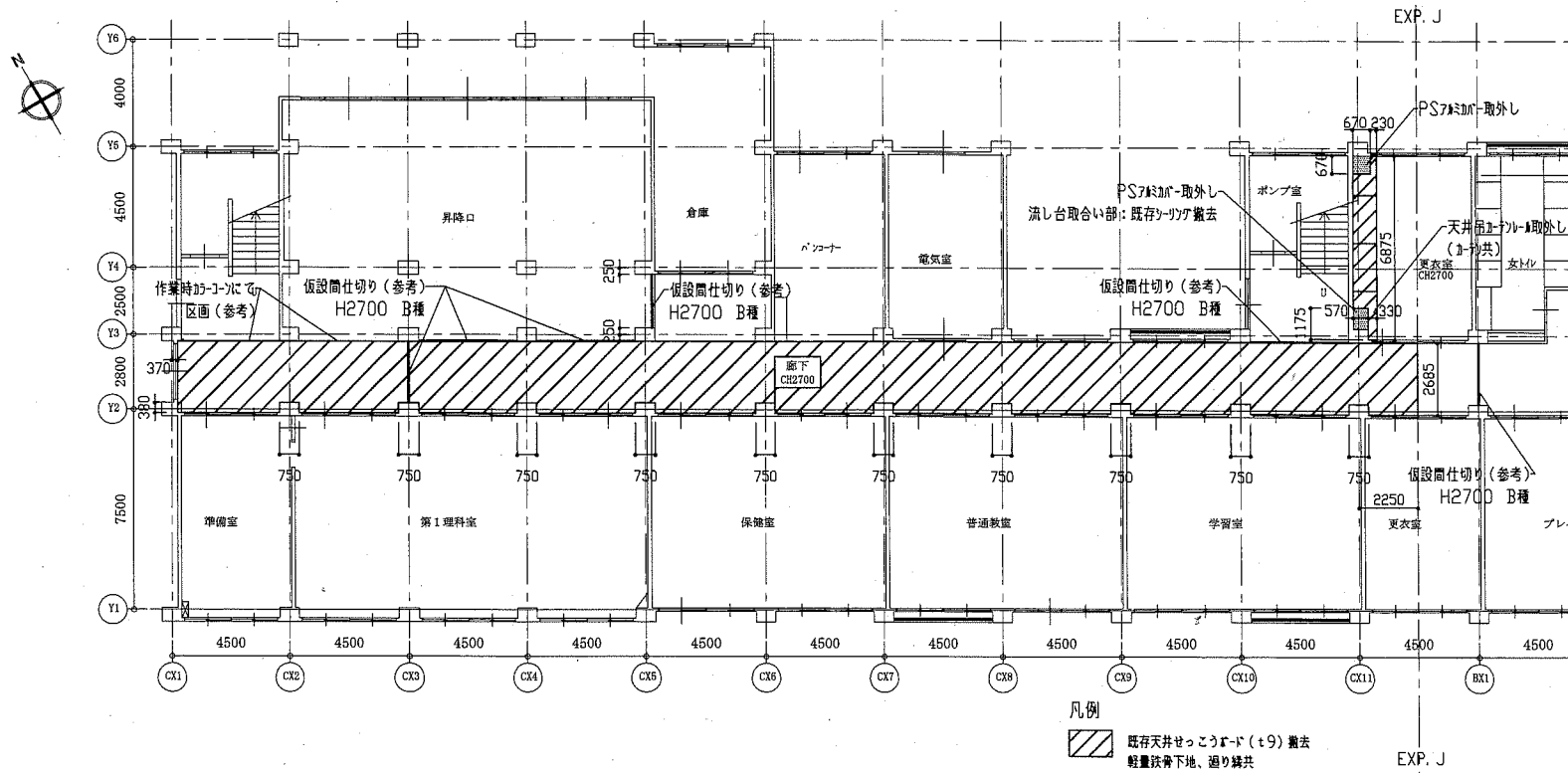
1階天井伏図 1/200
