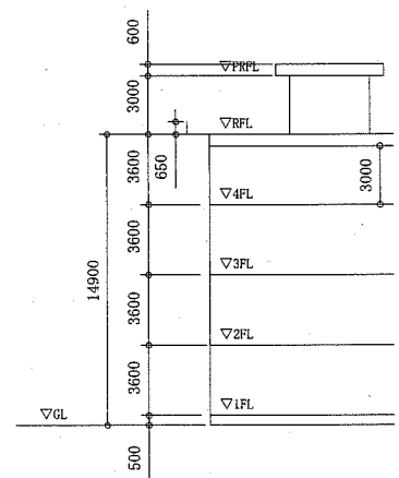
立面図 no scale
