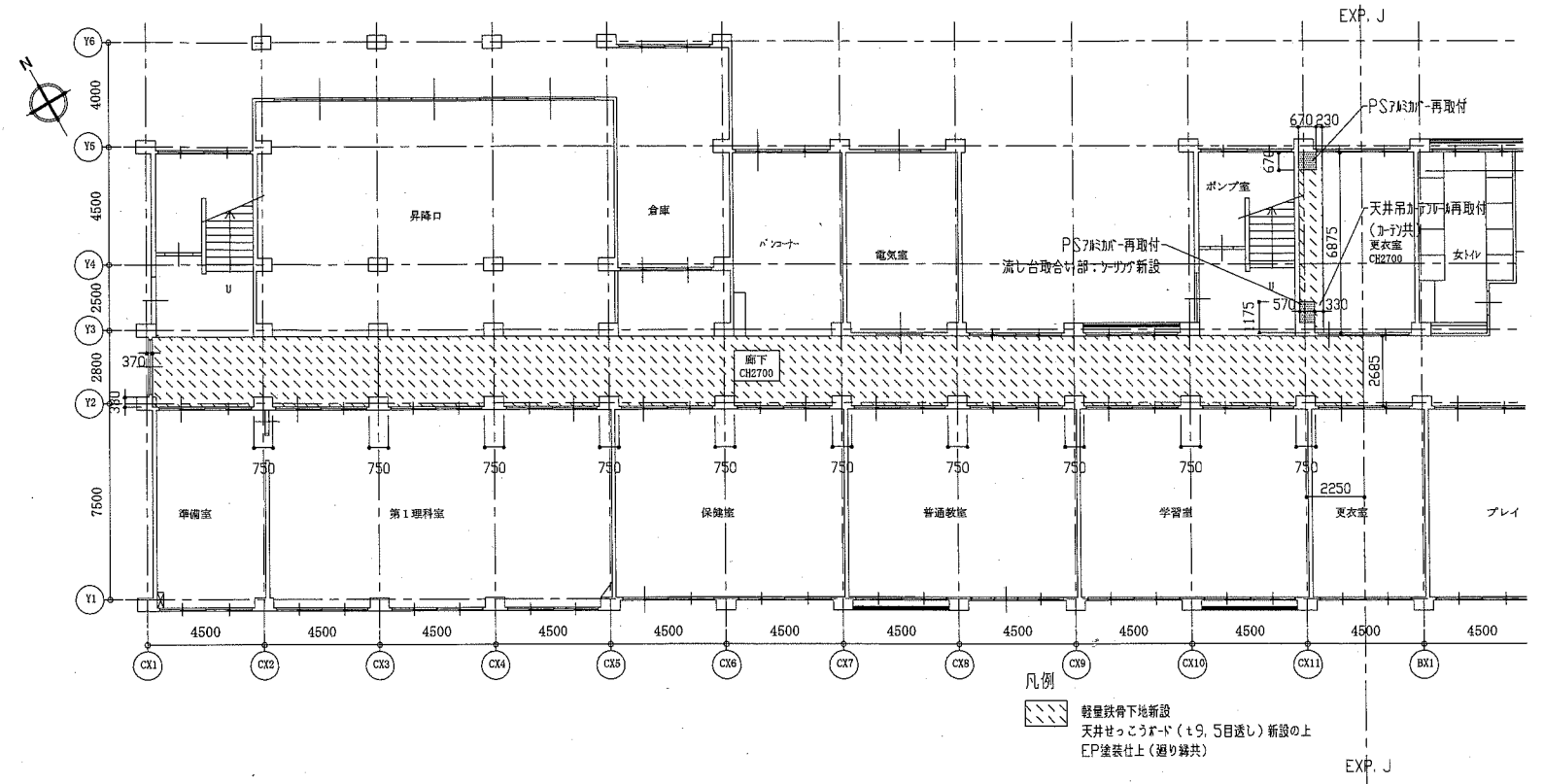
1階天井伏図 1/200
