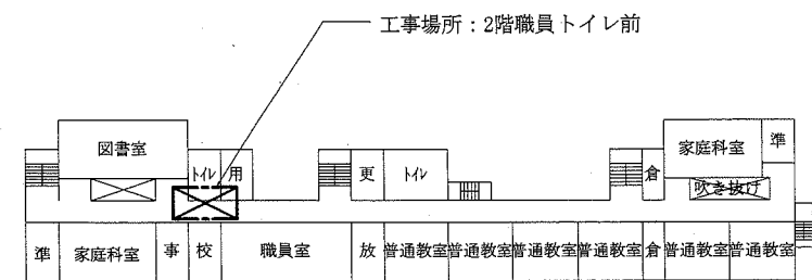
2階平面図 1:800
