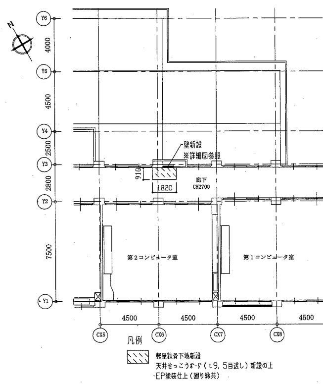
3階天井伏図 1/200
