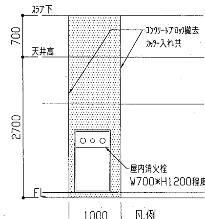
3階PSコンクリートアロワ-壁詳細図 1/50
