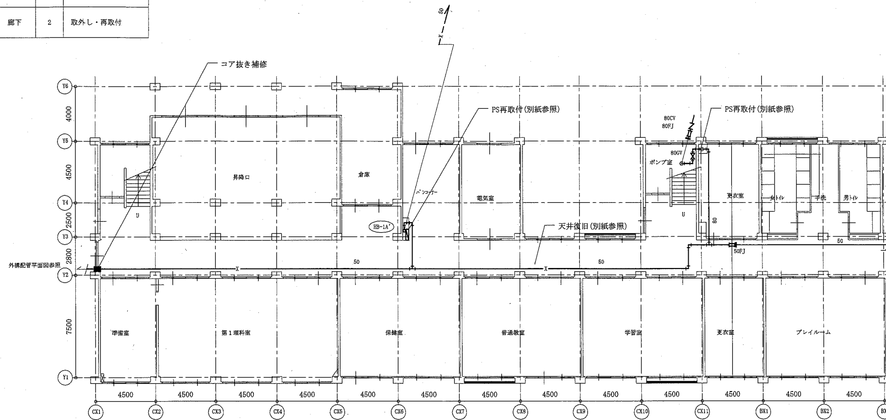
1階配管平面図(新設) 1:200
