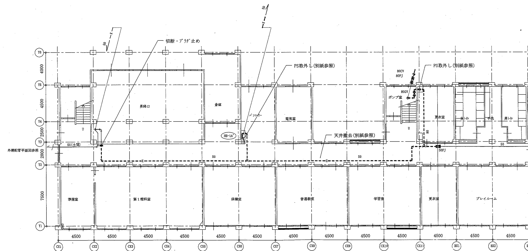
1階配管平面図(撤去) 1:200
