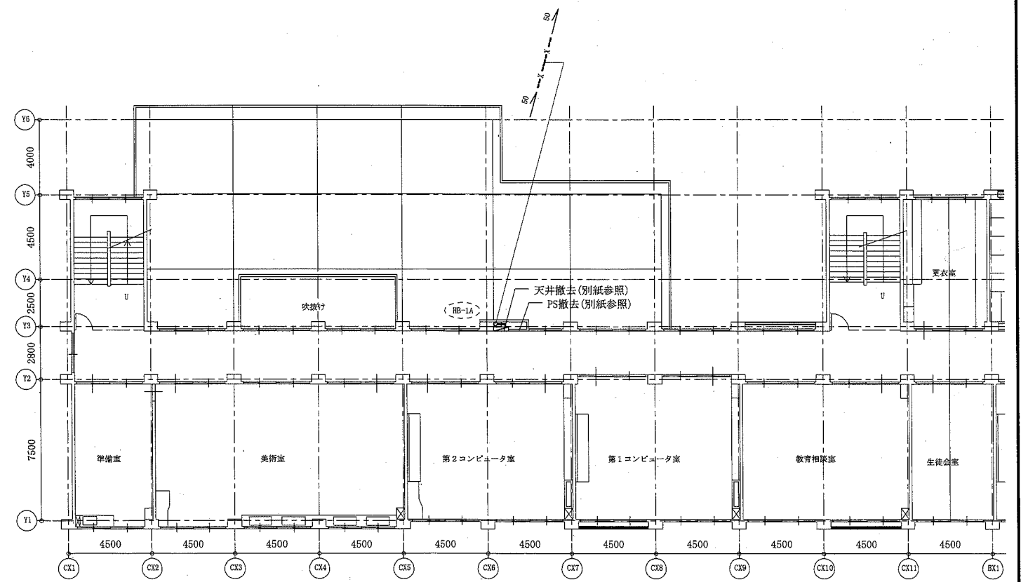
3階配管平面図(撤去) 1:200
