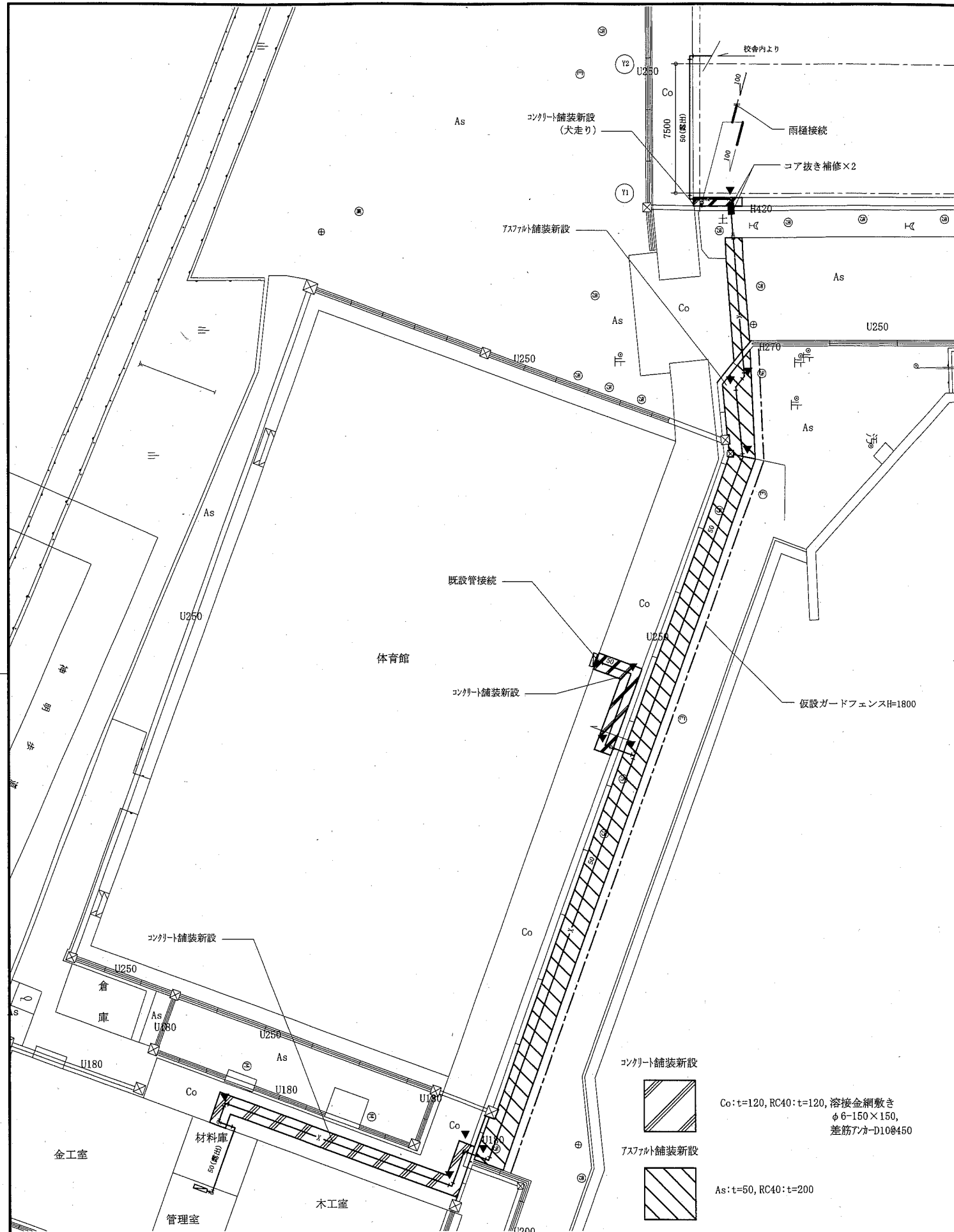
外構配管平面図(新設) 1:200 ▼:埋設表示ピン(頭はGLとフラットとする)
