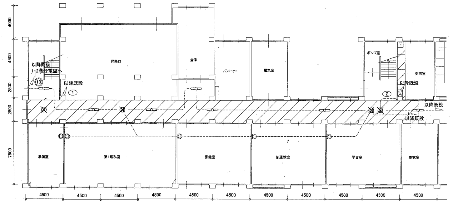
1階電気設備撤去図 1:200
