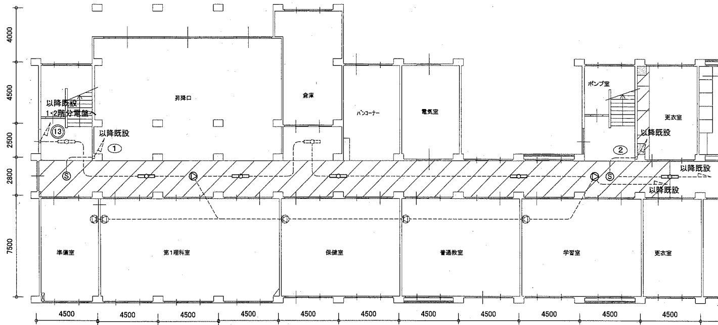
1階電気設備改修図 1:200
