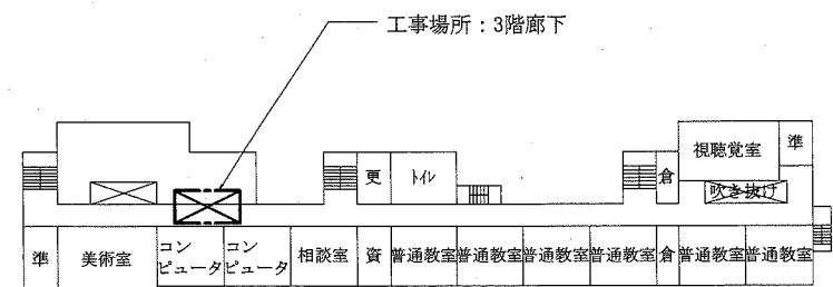
3階平面図 1:800
