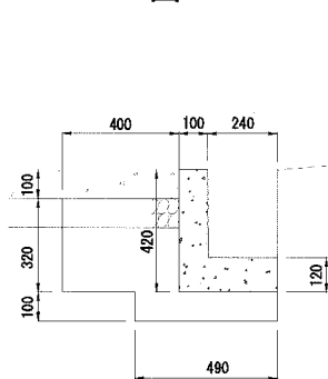
U型側溝とりこわし・床掘 図
