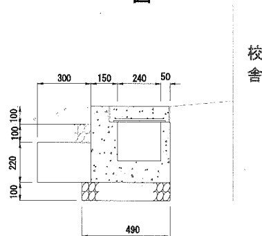
U型側溝埋戻し 図
