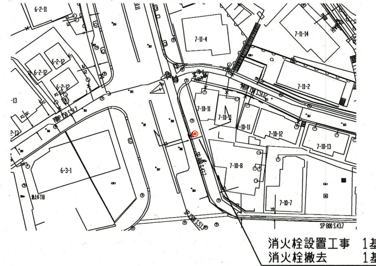
配管図
