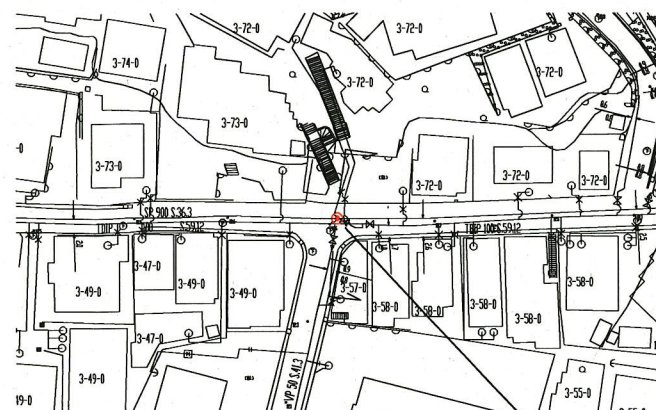
平面図 S=1/500
