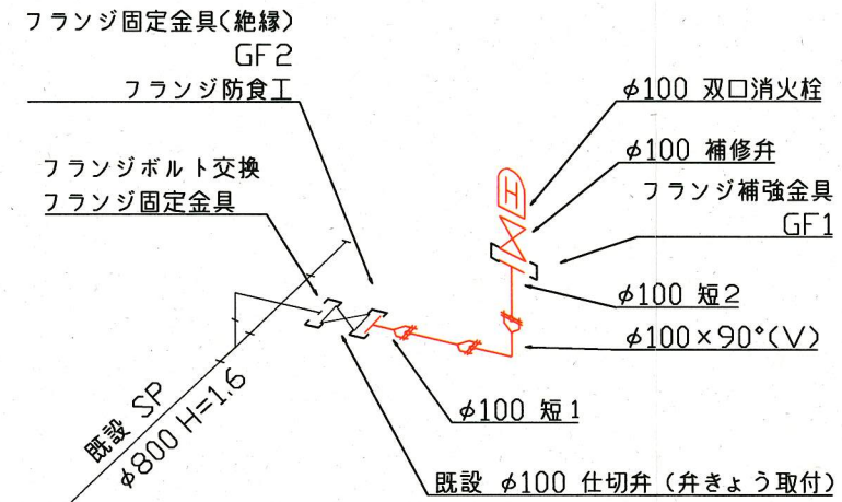
断面図 S=1/30
