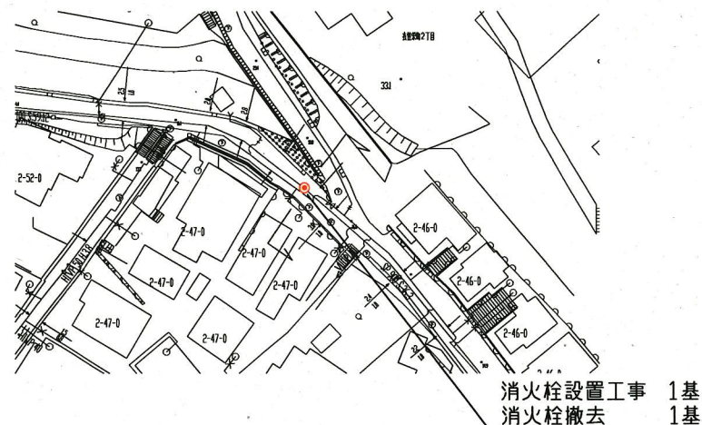
配管図
