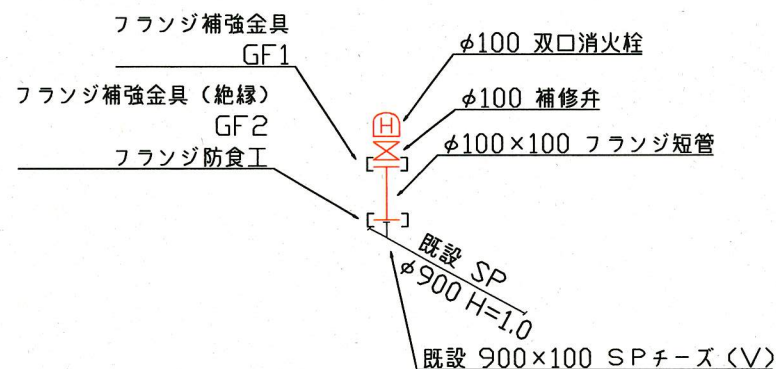
配管図
