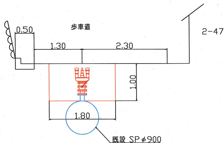
断面図 S=1/30
