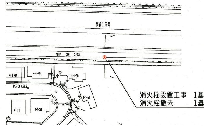
平面図 S=1/500
