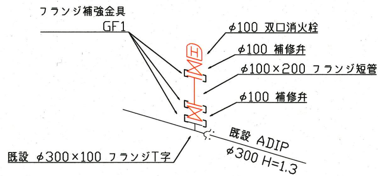
断面図 S=1/30
