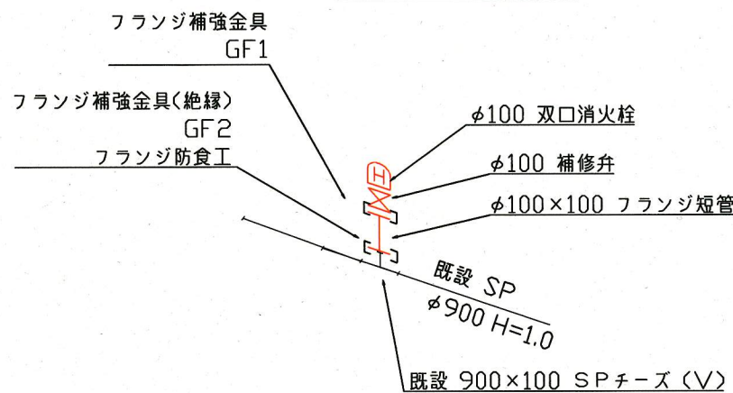
配管図
