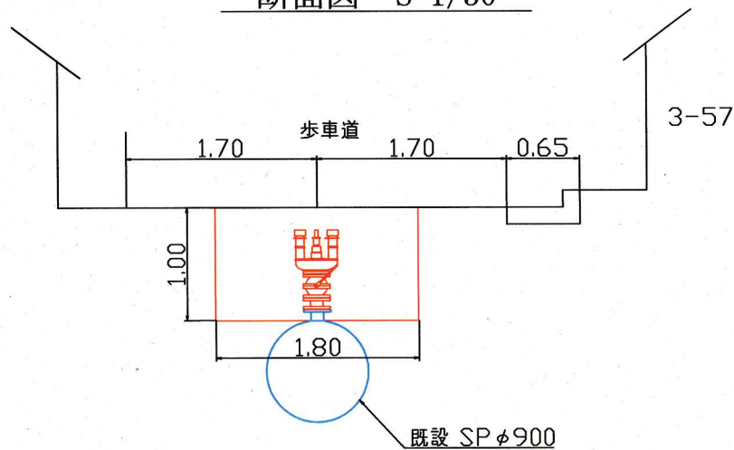
断面図 S=1/30
