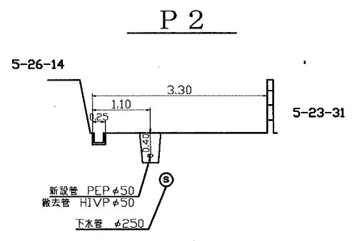
断面図 S=1/50
