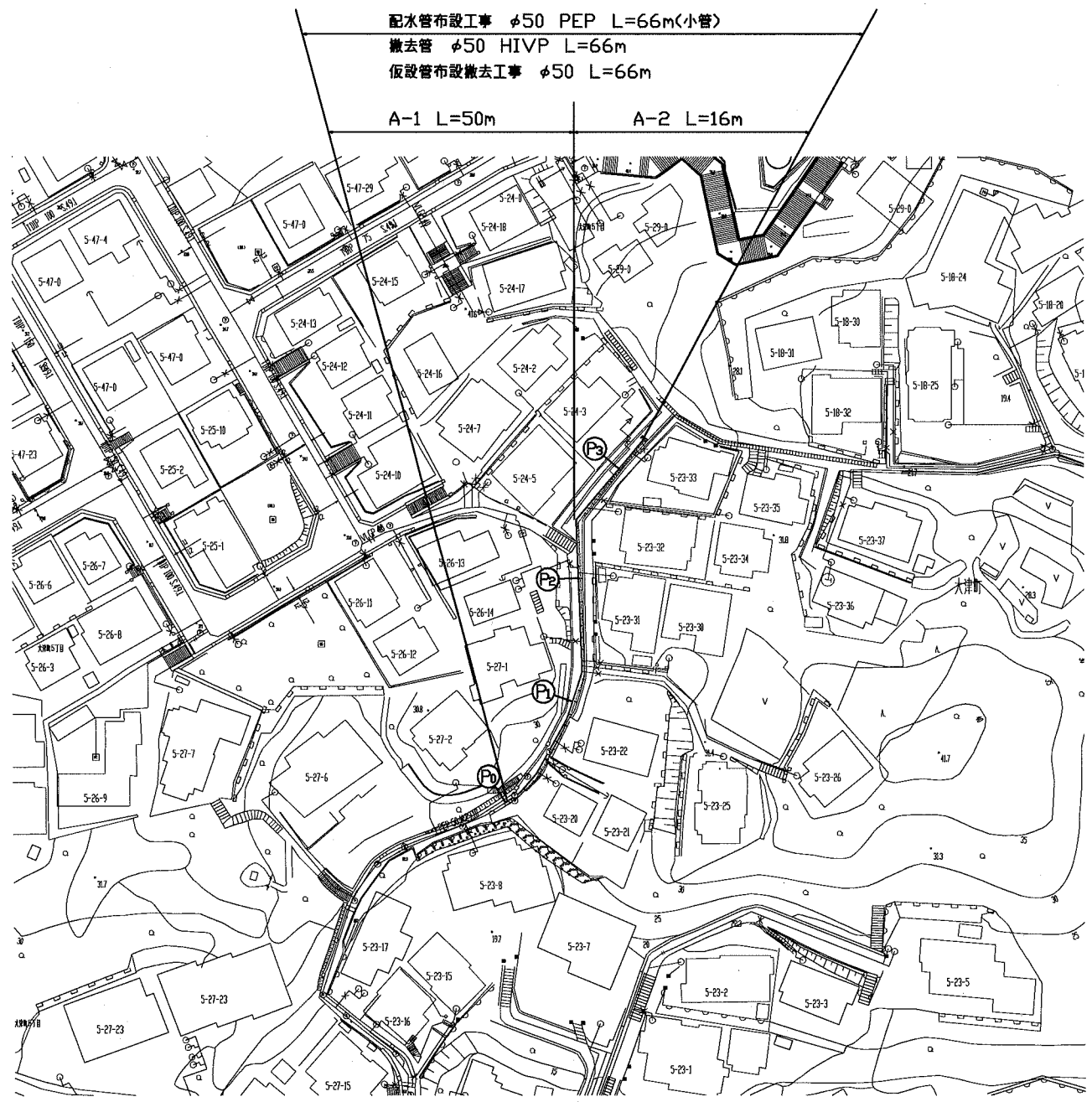
平面図 S=1/500
