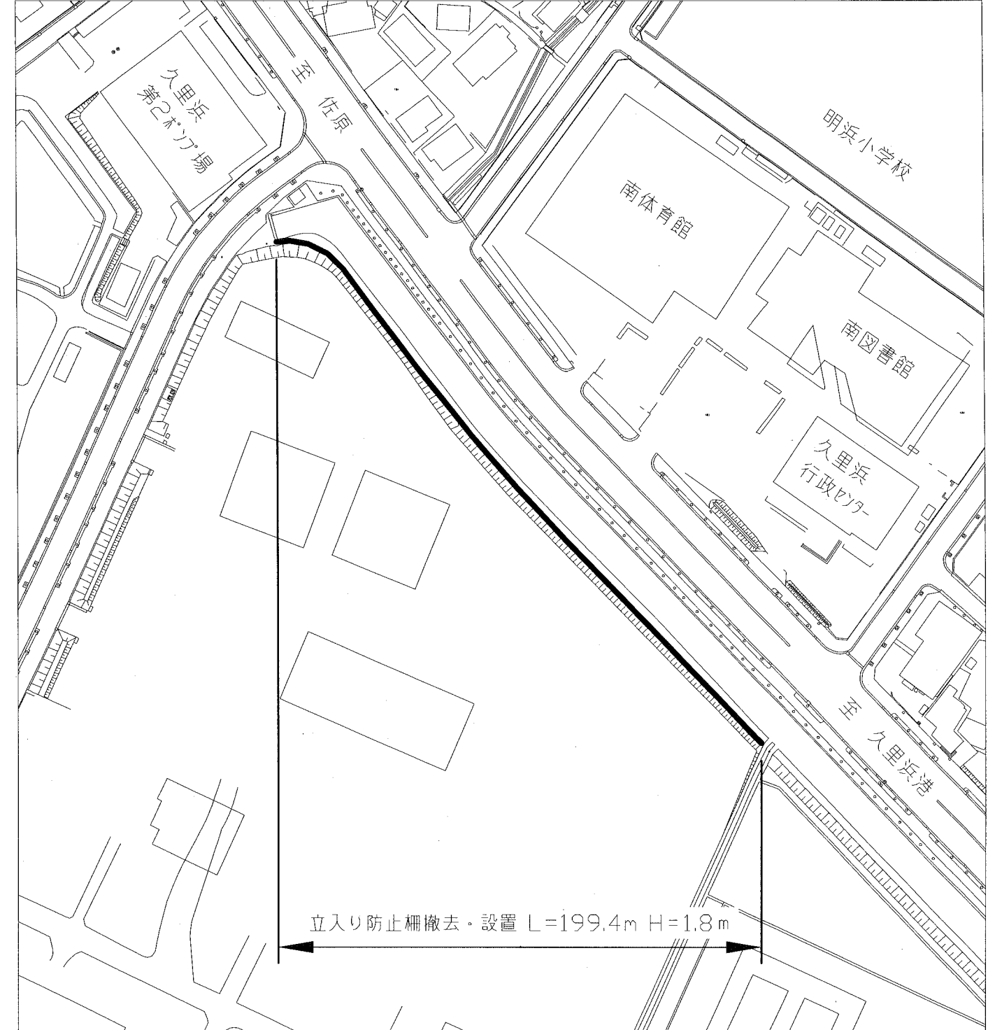
平面図 縮尺1:1500
