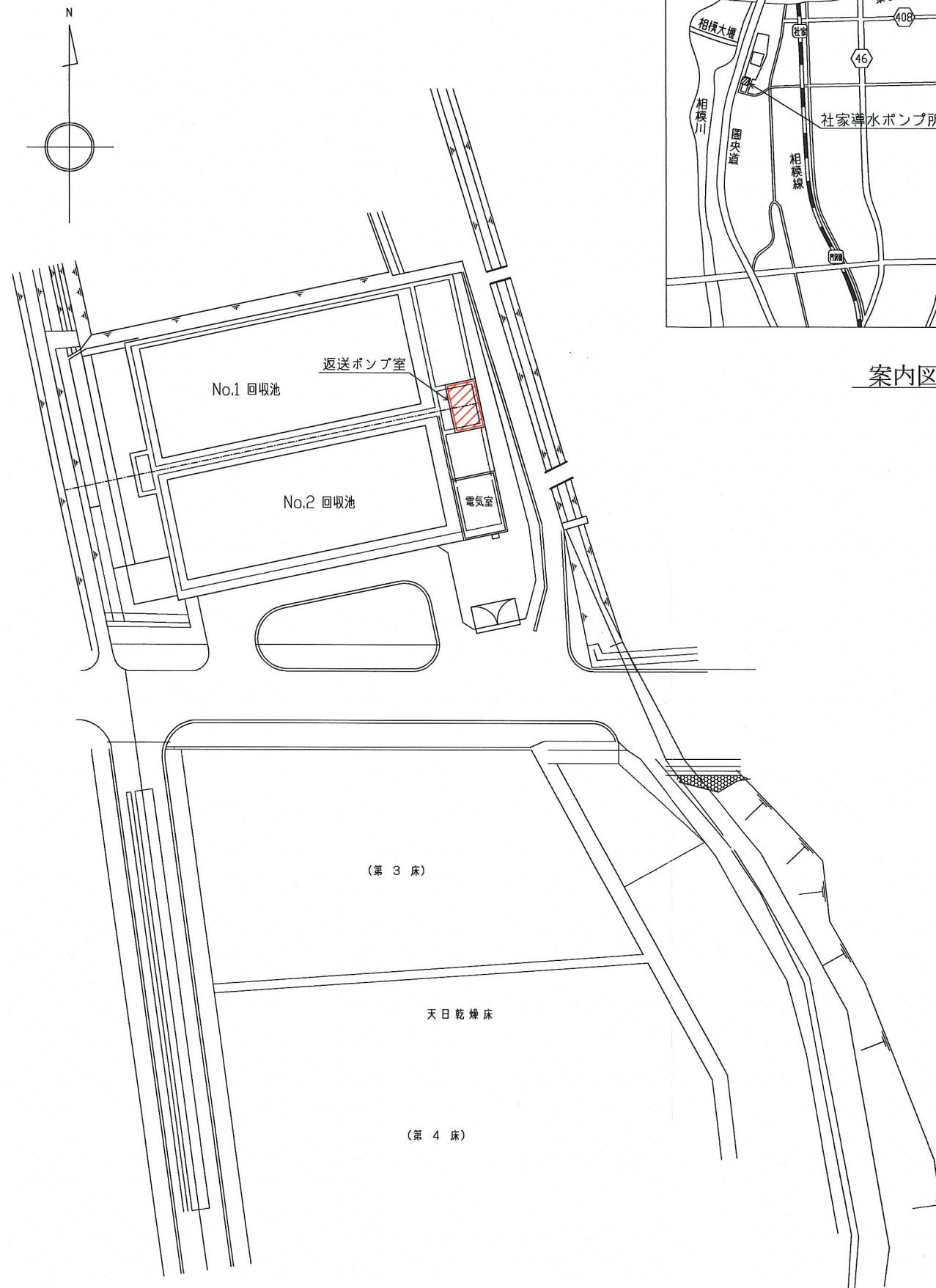
回収池平面図 S=NON
