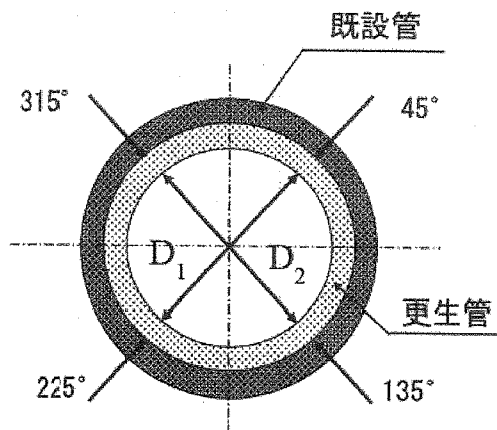
(図-1) 仕上り内径の測定位置 (参考)
