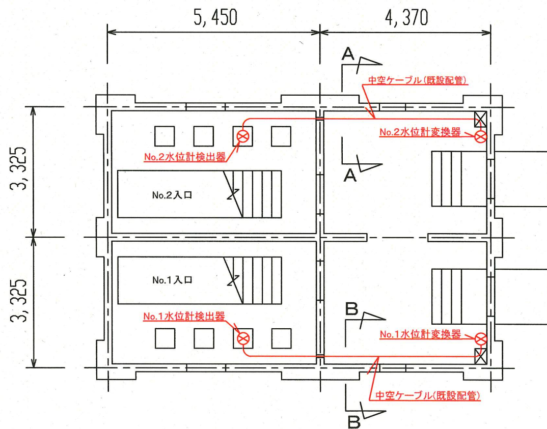
逸見2号配水池 排水管弁室 平面図 (S = 1/100)
