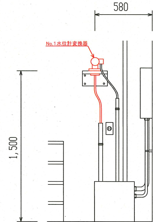
No.1水位計変換器 取付位置図 (S = 1/20) B - B 断面図
