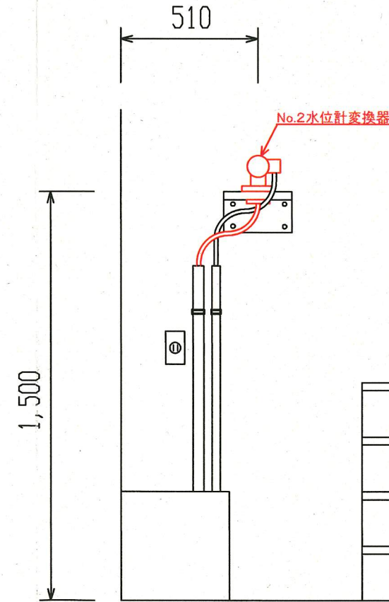
No.2水位計変換器 取付位置図 (S = 1/20) A - A 断面図
