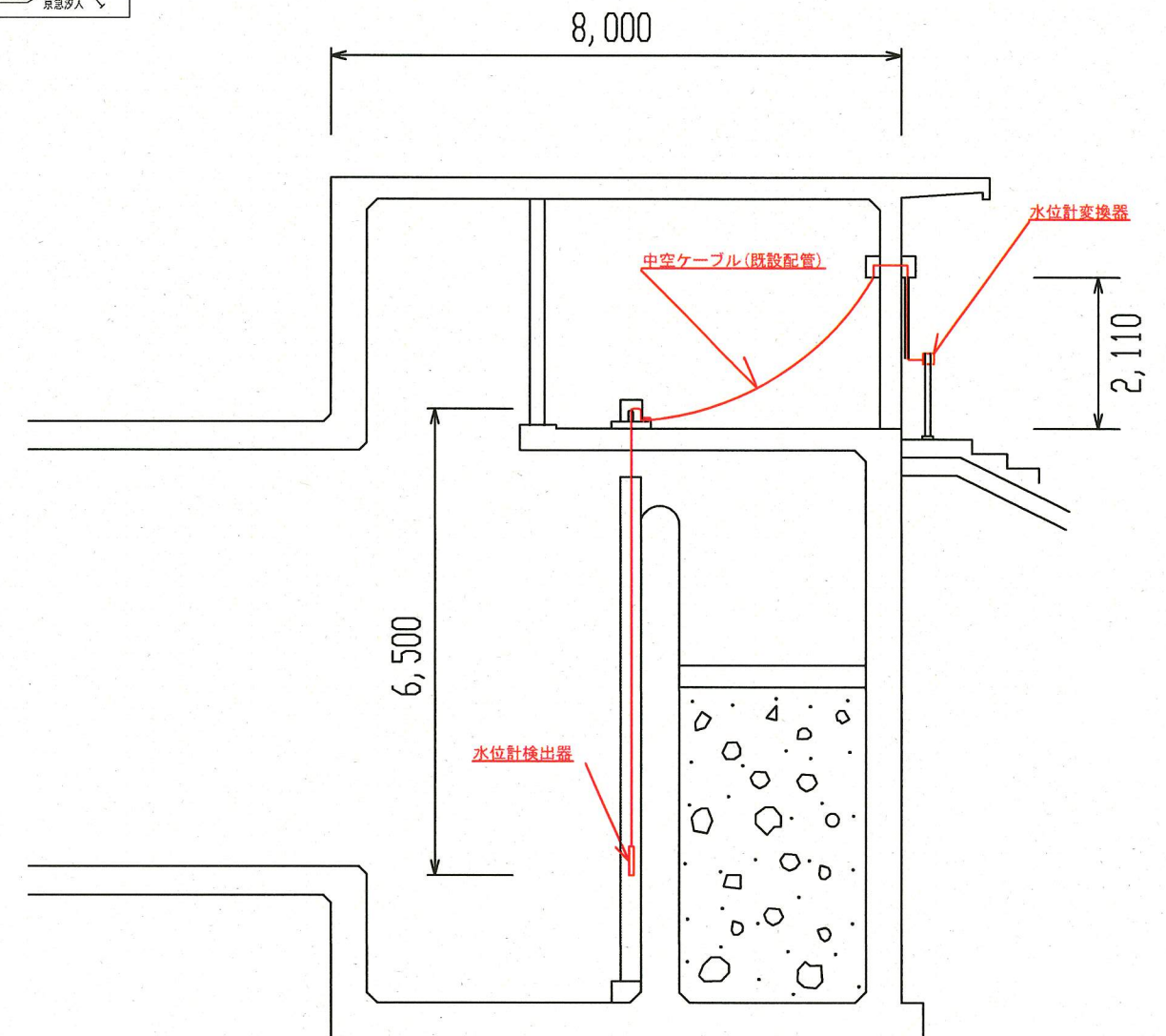
池上ずい道配水池 断面図 (S= 1/100)
