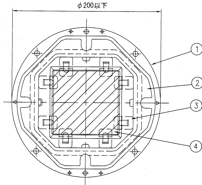
平面図
